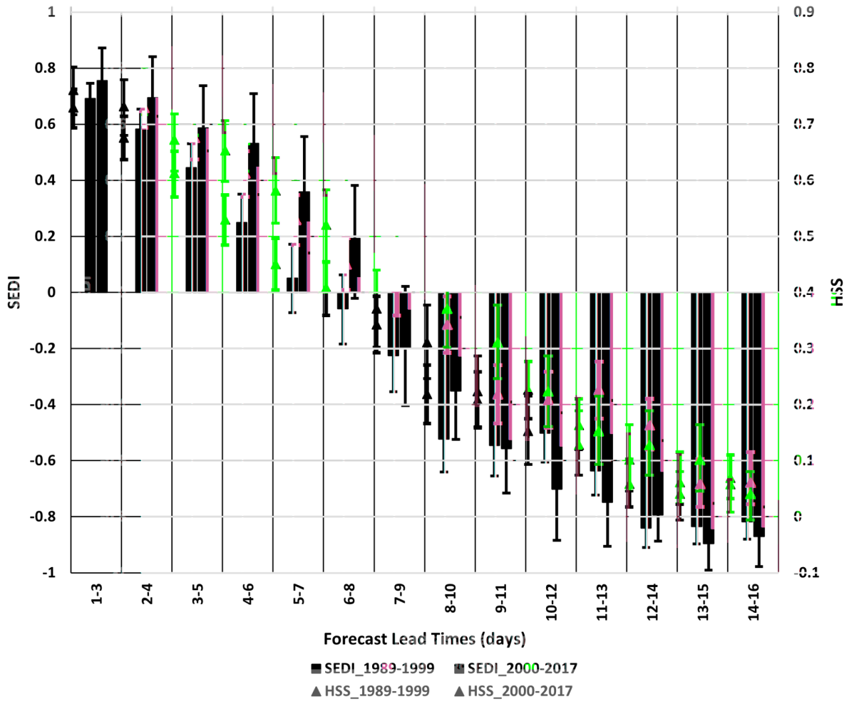
GEFSv12 Yuba Dec- Mar 1989-1999 vs 2000-2017
