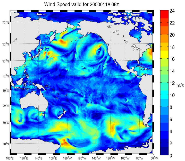
Fig. 3.2 : CFSRR winds valid 2000/01/18 06z.
