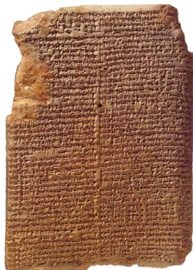
もっとも古い星座の教科書『ムル・アピン』
