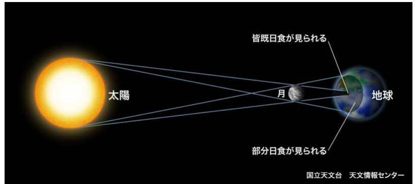
日食がおこるしくみ（国立天文台 天文情報センター）
