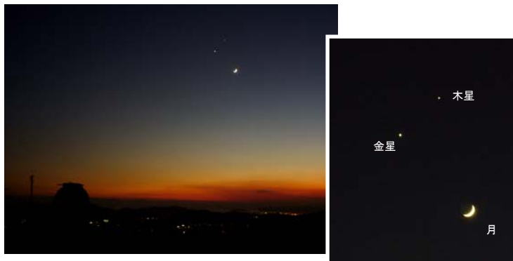
2008年12月1日、夕方の西空に見られた金星と木星、月の接近 (撮影: 本田敏志 氏)
