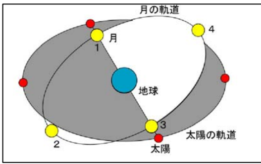
図4. 月の通り道(白道)と太陽の通り道(黄道)
