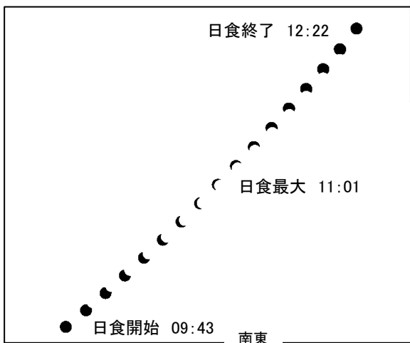
図6. 浅口市での日食の様子
