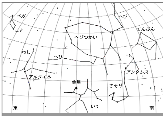
図. 2月中旬午前6時頃の空(浅口市) 3月1日には、金星と細い月が接近する。
