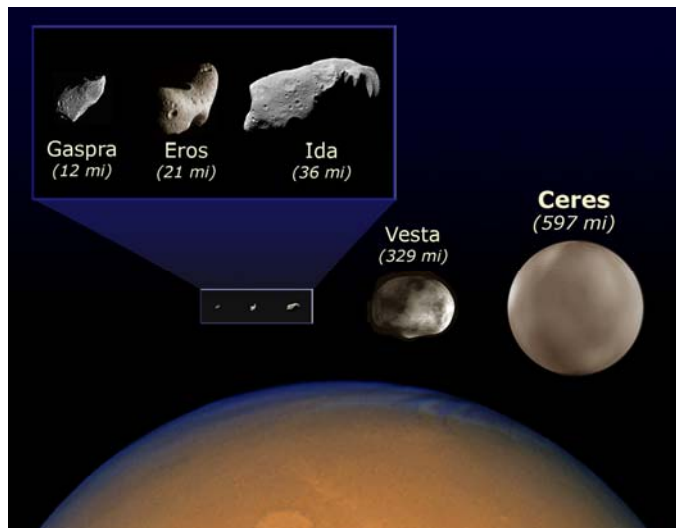
図. 主な小惑星と火星の大きさの比較 ©NASA, ESA, and A. Feild (STScI)
