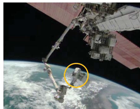
船外活動(EVA)を行う米国人宇宙飛行士をロボットアームの先端に乗せ、熱制御系ポンプを交換を支援
