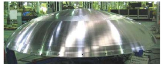
(注) 写真は実機大工作試験での機械加工後のもの
