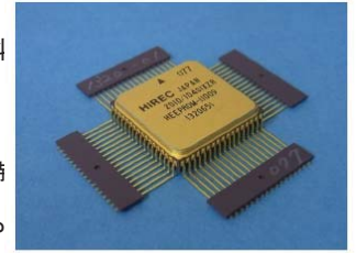
4Mbit EEPROM外観
