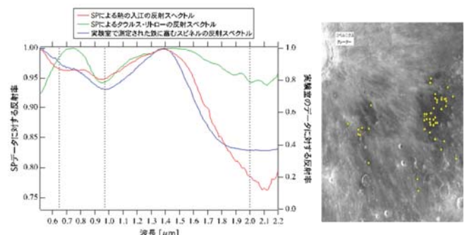
左図: 分光データで測定された特殊な反射スペクトルデータ(赤線)。従来測定されていたのは緑線とは傾向が異なることが分かる。 右図: 特殊な反射スペクトルの検知地点(黄色)がダークマントル堆積物(黒っぽい領域)に集中していることが分かる。
