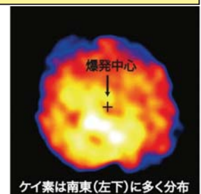
図: 超新星残骸がケイ素の輝線で観測した画像
