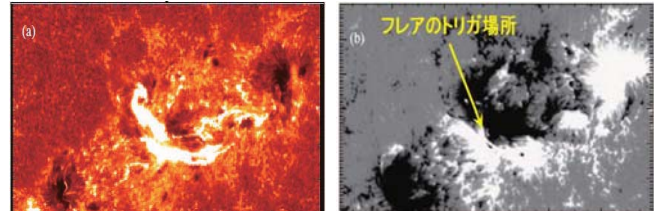
左図: 「ひので」で観測した彩層のフレア画像 右図: 光球面の磁場データ。彩層画像からわかるフレアのトリガ場所での磁場構造を同定。
