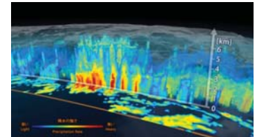
(a) DPRによる降水の三次元分布
