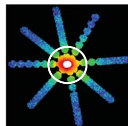
図: 「すざく」がとらえたペルセウス座銀河団のX線画像(中心円は、すざく以前に元素量測定が可能だった範囲)
