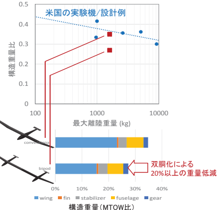
超高アスペクト比翼の設計検討 (双胴化による重量低減効果の確認)
