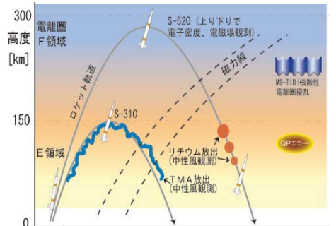
図:S-310-42号機(下曲線)とS-520-27号機(上曲線)の飛行経路・高度と観測対象(E・F領域で発生する各種擾乱)、観測手法(TMA放出等)の関係図
