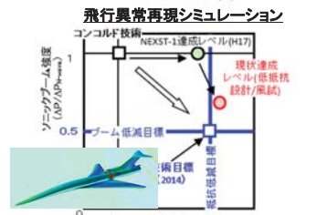
小型超音速機概念形状の性能推算
