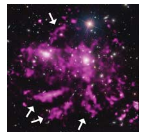
図：かみのけ座銀河団の中に見つかった、X線で輝く巨大な腕
