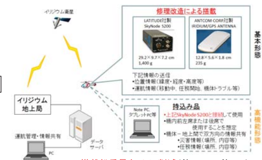
搭載総重量を1/4に削減(約20kg→約5kg) 搭載性向上型D-NET機上機器の開発
