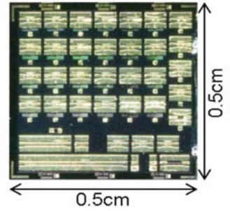
試作MEMSスイッチ (10種類32個)
