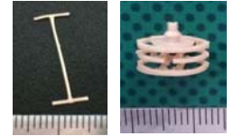
宇宙用タグピンと新スペーサ
