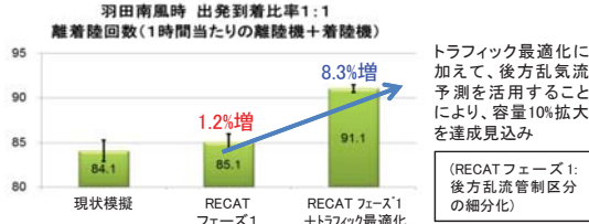
高密度運航シミュレーションの結果例
