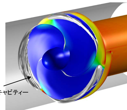
インデューサキャビテーション解析結果例 (キャビティと翼面上圧力分布)
