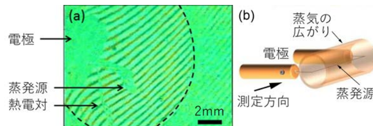
S-520-28実験結果の例。蒸発した鉄が核生成する際のガスの温度と濃度を独自開発の光学系によりその場測定した。(a) 得られた画像、(b) 測定方法の概略図。鉄蒸気が蒸発源から同心円状に広がりながら冷えて(左図の破線の内側)、固体微粒子になった。
