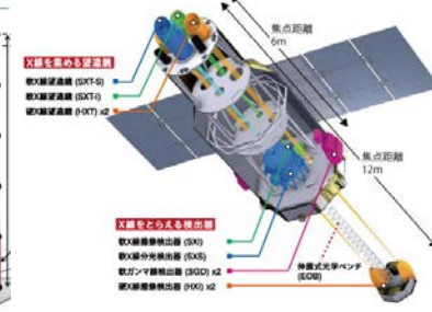
ASTRO-H 6台の観測機器の配置
