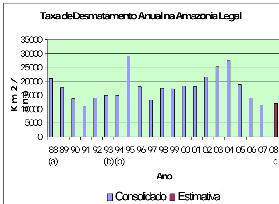
Figura 5.4 – Evolução da taxa de desmatamento de 1988 a 2008 (a: média 1977 a 1988; b: média 1992 a 1994; c: estimativa)
