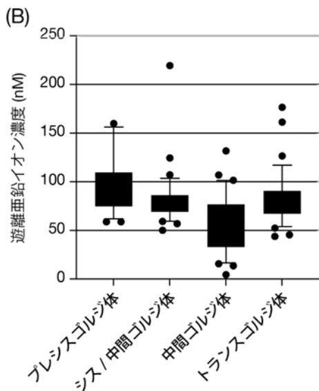
図 1. ゴルジ体遊離亜鉛イオン濃度測定 (A) ゴルジ体の各層板に局在する様々な HaloTag 融合タンパク質を作製し、ZnDA-1H をそのゴルジ層板に特異的に局在させ、生細胞亜鉛イメージングを行った。(B)各ゴルジ層板における遊離亜鉛イオン濃度の定量値。
