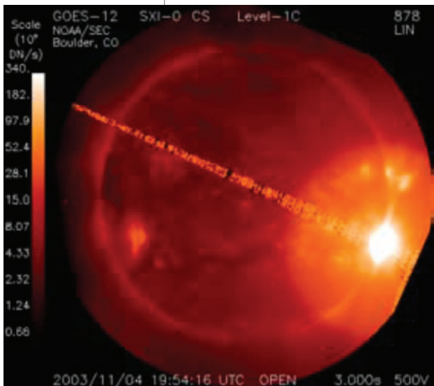
Solar Flare
