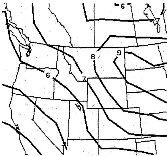
B) MSLP (mb)
