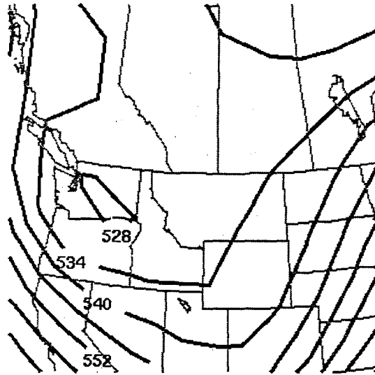
A) 500MB Heights (dm)
