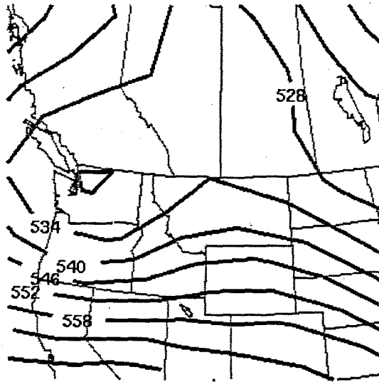
A) 500MB Heights (dm)
