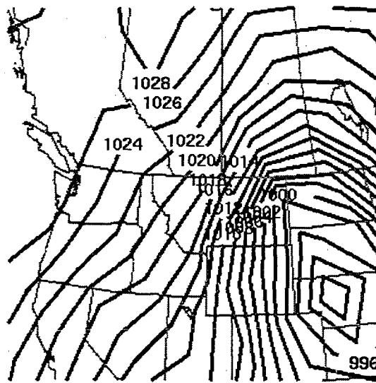
B) MSLP (mb)
