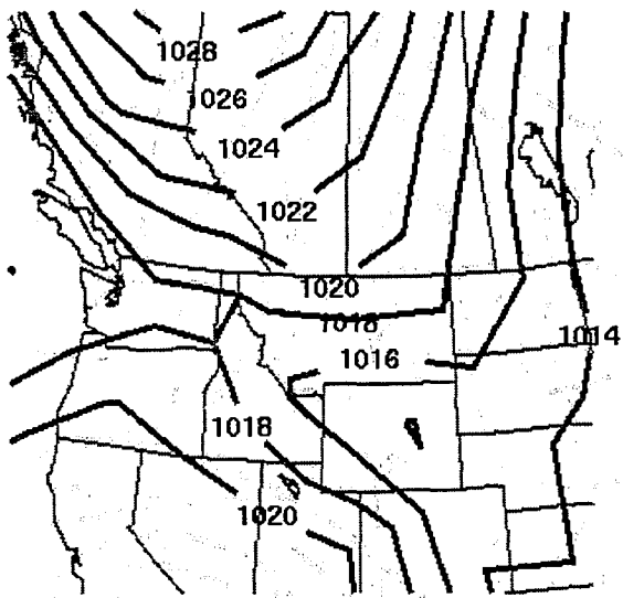
B) MSLP (mb)
