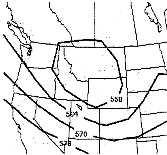
A) 500MB Heights (dm)
