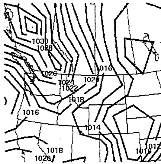
B) MSLP (mb)
