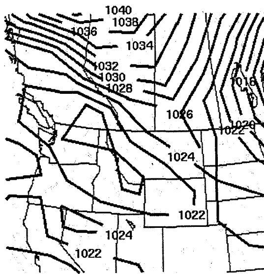
B) MSLP (mb)
