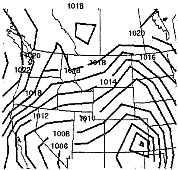
B) MSLP (mb)
