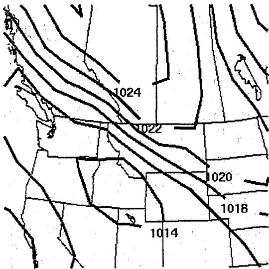
B) MSLP (mb)
