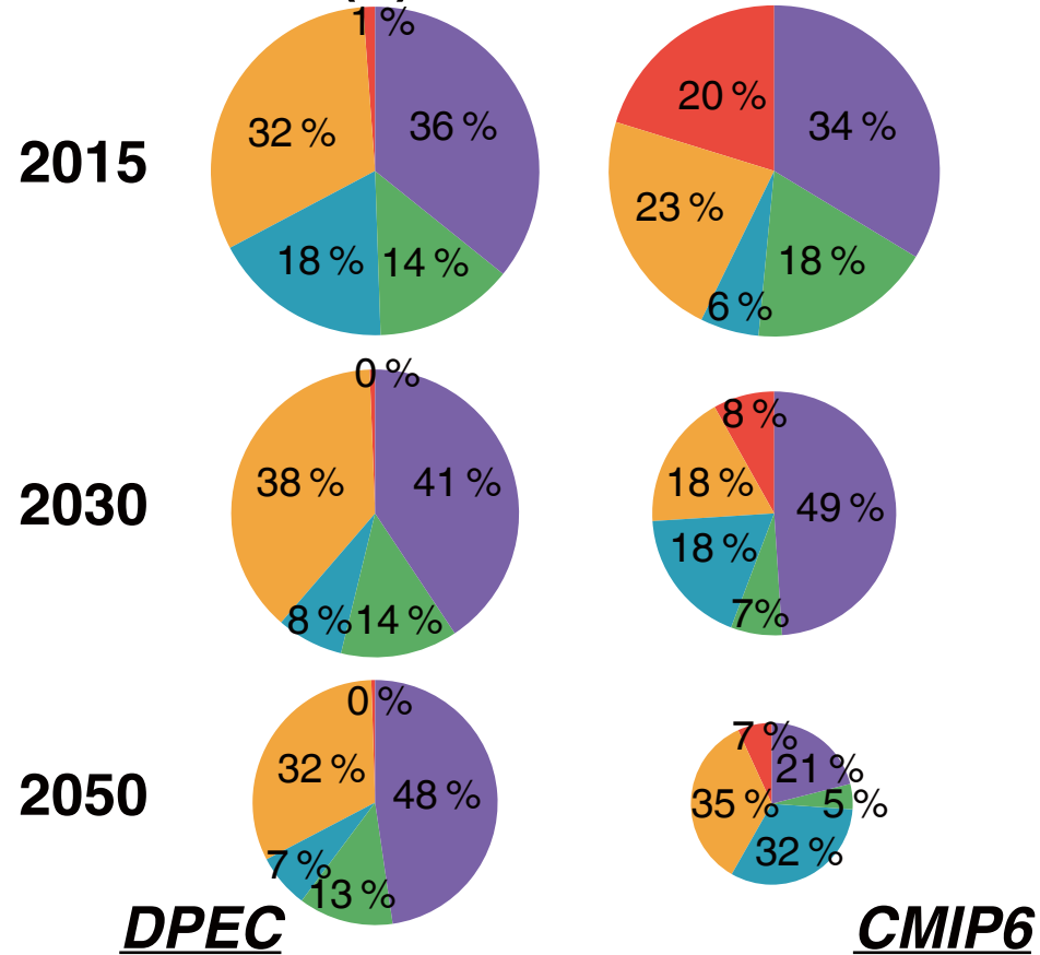
(d) NMVOCs
