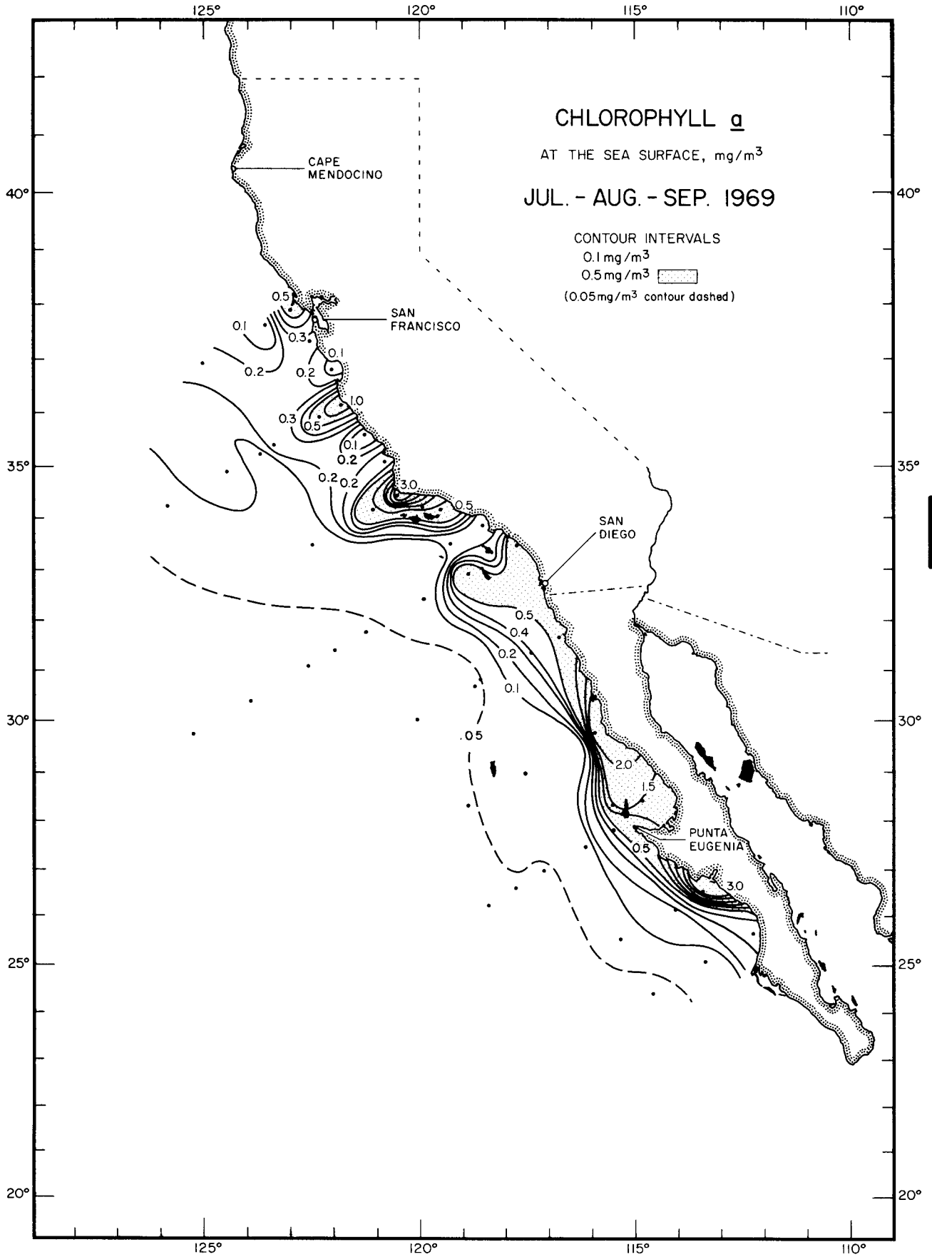
CHLOROPHYLL a SURFACE JUL. - AUG. - SEP. 1969
