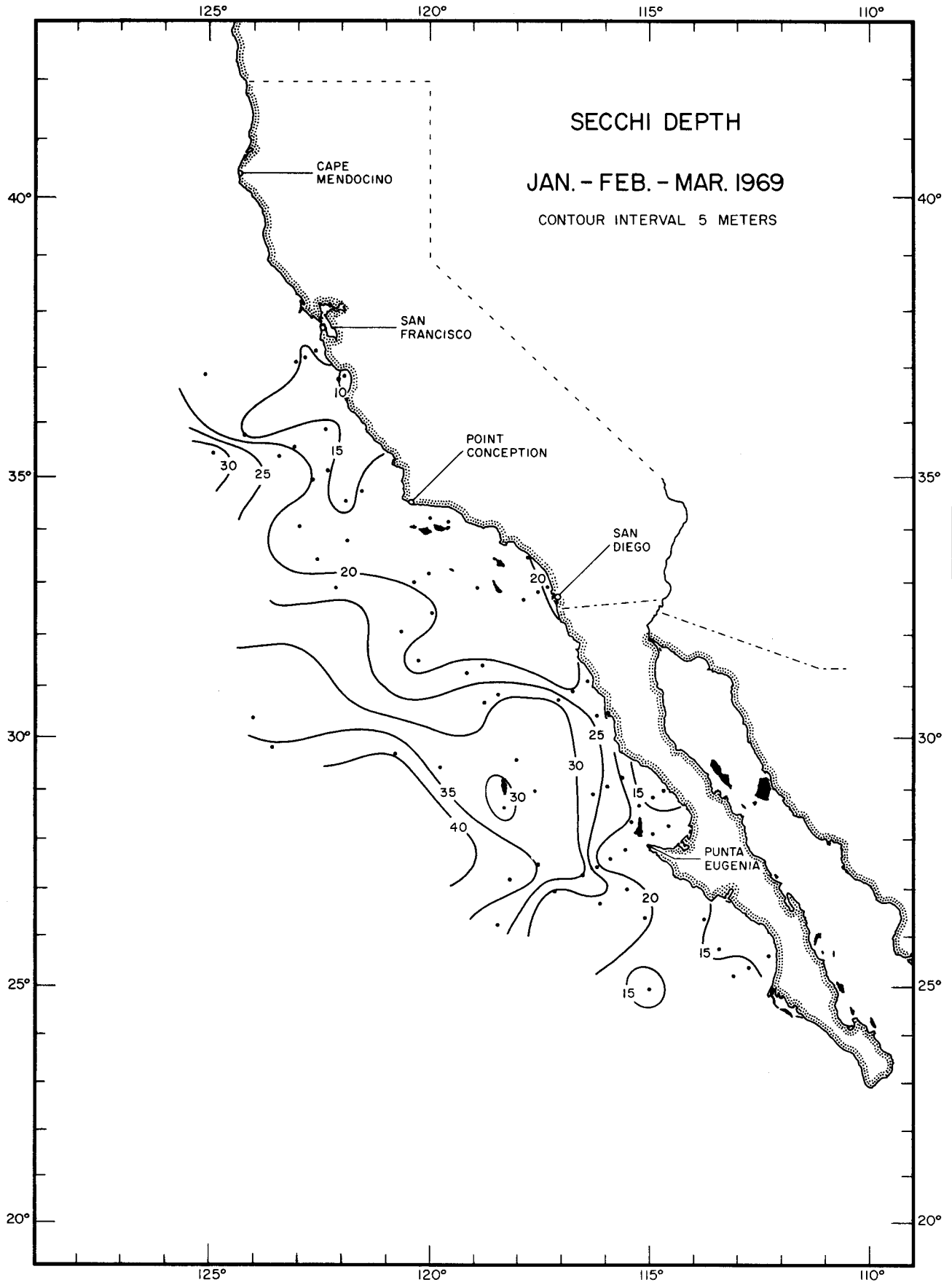
SECCHI DEPTH JAN. - FEB. - MAR. 1969
