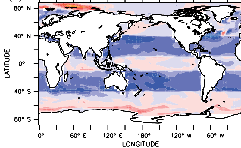
RCP8.5_AOA_ST
