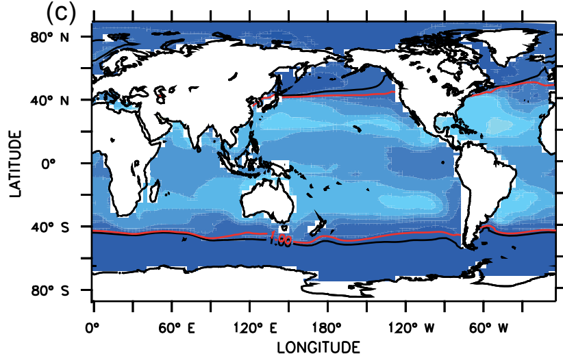
RCP8.5_AOA_ST
