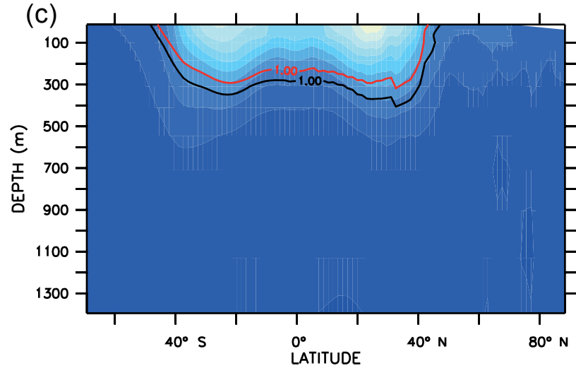
RCP8.5_AOA_ST
