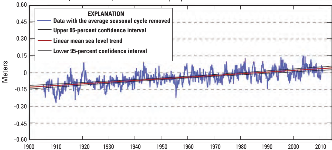
D. Nawiliwili, Hawaii 1.53 +/- 0.59 millimeters per year
