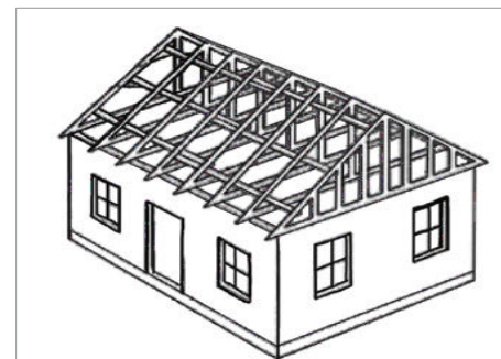
Figura 4-2. Treliças são construídas com um pico na linha de cumeeira da casa. As treliças no final da casa formam um padrão em forma de A conhecido como extremidade de empena. Durante um furacão, a extremidade da empena está sujeita a grandes forças do vento e pode tombar, derrubando as outras treliças de forma dominó. Fonte: Brochura Contra o Vento 247 da FEMA.
