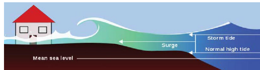
Figura 2-2. Representação de ressacas. Crédito da imagem: NOAA/ The Comet Program.
