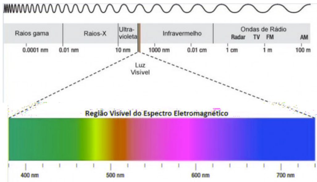
Figura – Espectro Eletromagnético (Fonte: http://know.net/cienciasexactas/fisica/espectroelectromagnetico )
