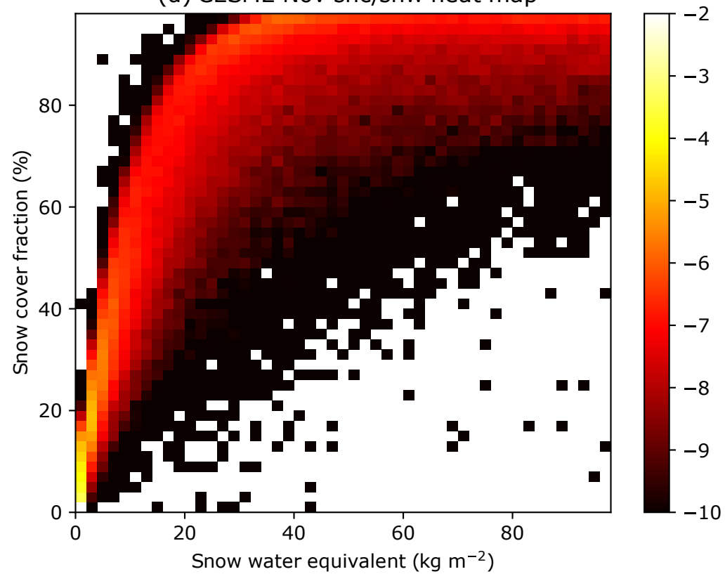
(d) CESM2 Nov snc/snw heat map
