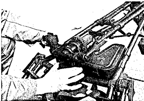
Oberlafette lösen
