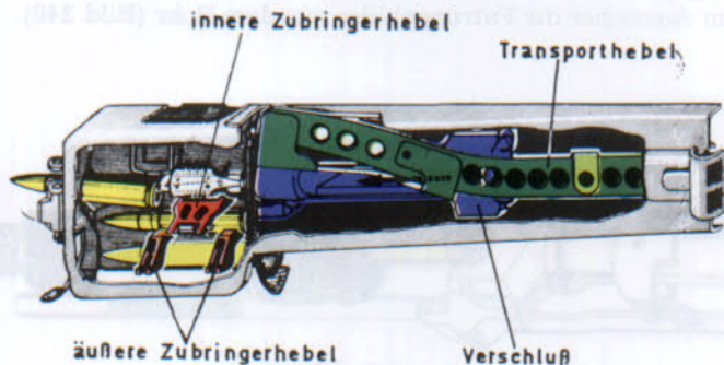
Transporthebel bei beginnendem Verschußvorlauf
