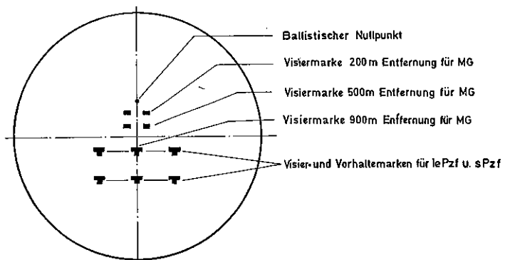
Strichbild des Bildverstärker-Zielfernrohrs
