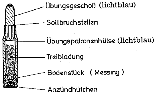
Aufbau einer Übungspatrone 7,62 mm × 51 DM18
