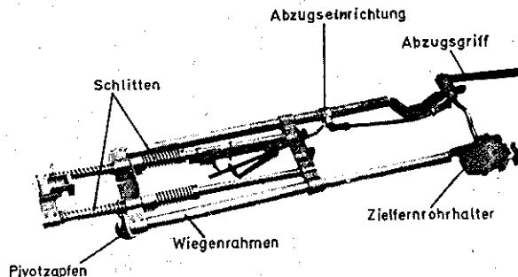
Oberlafette mit Wiegenrahmen, Schlitten und Abzugseinrichtung
