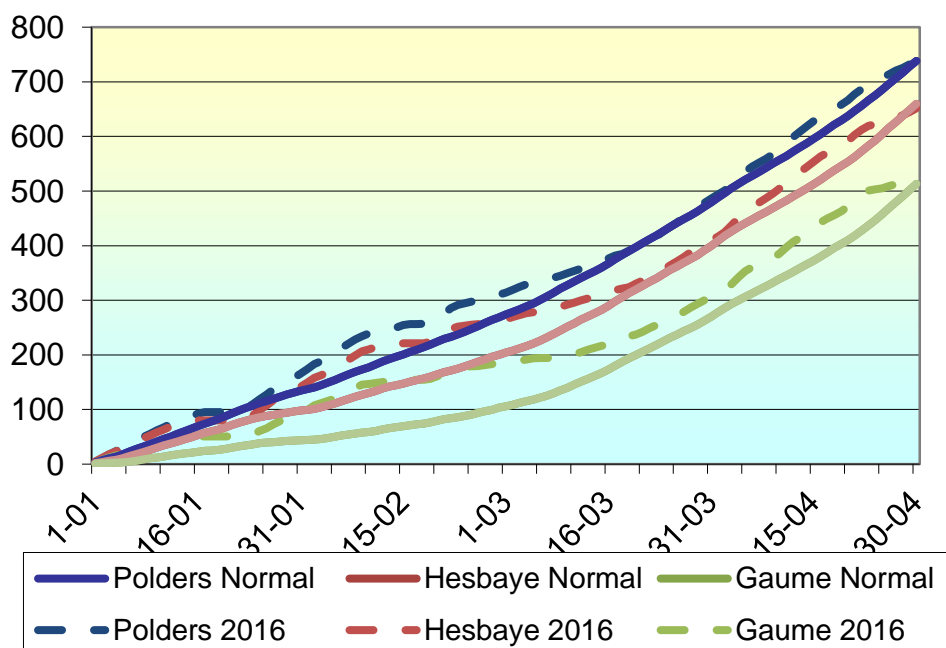
Fig. 2 : Evolution des sommes des températures (degrés.jours en base 0°C) en 2016 et en situation normale pour trois régions du nord, centre et sud du pays.
