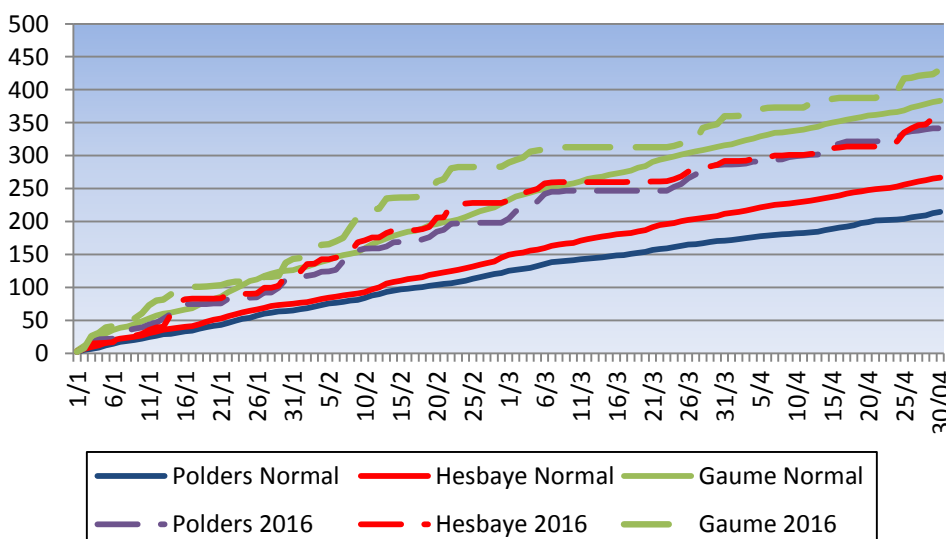
Fig. 3 : Evolution des précipitations cumulées en 2016 et en situation normale pour trois régions du nord, centre et sud du pays.
