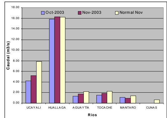
Gráfico 24. Niveles Medios Mensuales de la Zona Centro de la Vertiente del Atlántico
