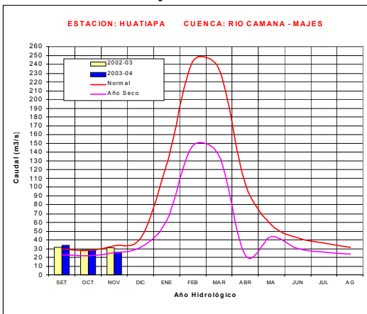
Gráfico 11. Caudal medio mensuales del año hidrológico 2002-2003, 2003-2004, año promedio o normal y año seco promedio del río Camaná - Majes
