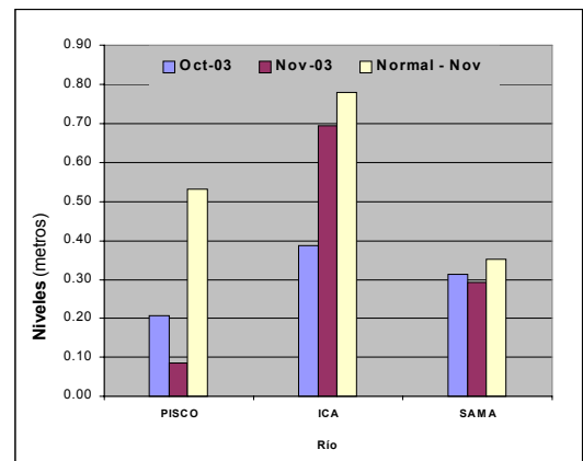
Gráfico 12. Niveles Medios Mensuales de la Vertiente del Pacífico Zona Sur por Cuencas
