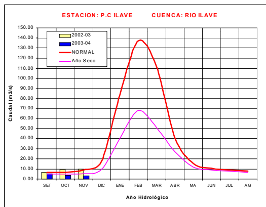
Gráfico 16. Caudal medio mensual del año hidrológico 2002-2003, 2003-2004, año promedio o normal y año seco promedio del río Ilave
