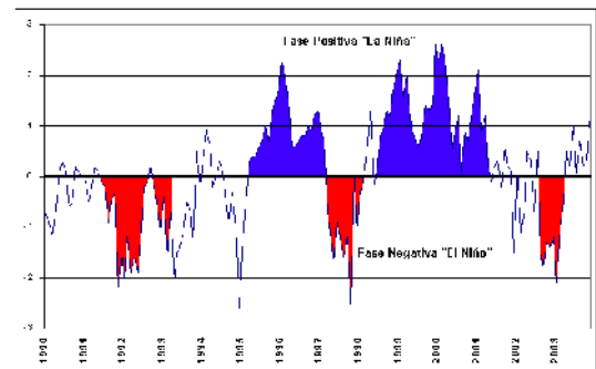
Figura 6. Índice de Radiación de Onda Larga
