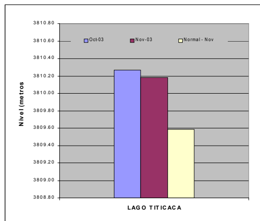
Gráfico 17. Niveles Medios Mensuales del Lago Titicaca
