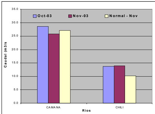
Gráfico 10. Caudales Medios Mensuales de la Vertiente del Pacífico Zona Sur por cuencas
