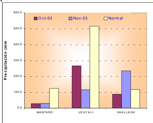
Gráfico 23. Precipitación Mensual de la Zona Centro de la Vertiente del Atlántico zona Centro por cuencas
