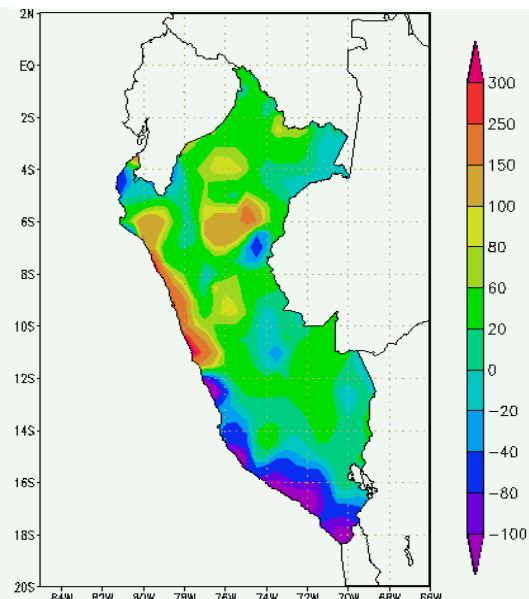
Mapa 3. Anomalías de la precipitación (%) Diciembre 2003
