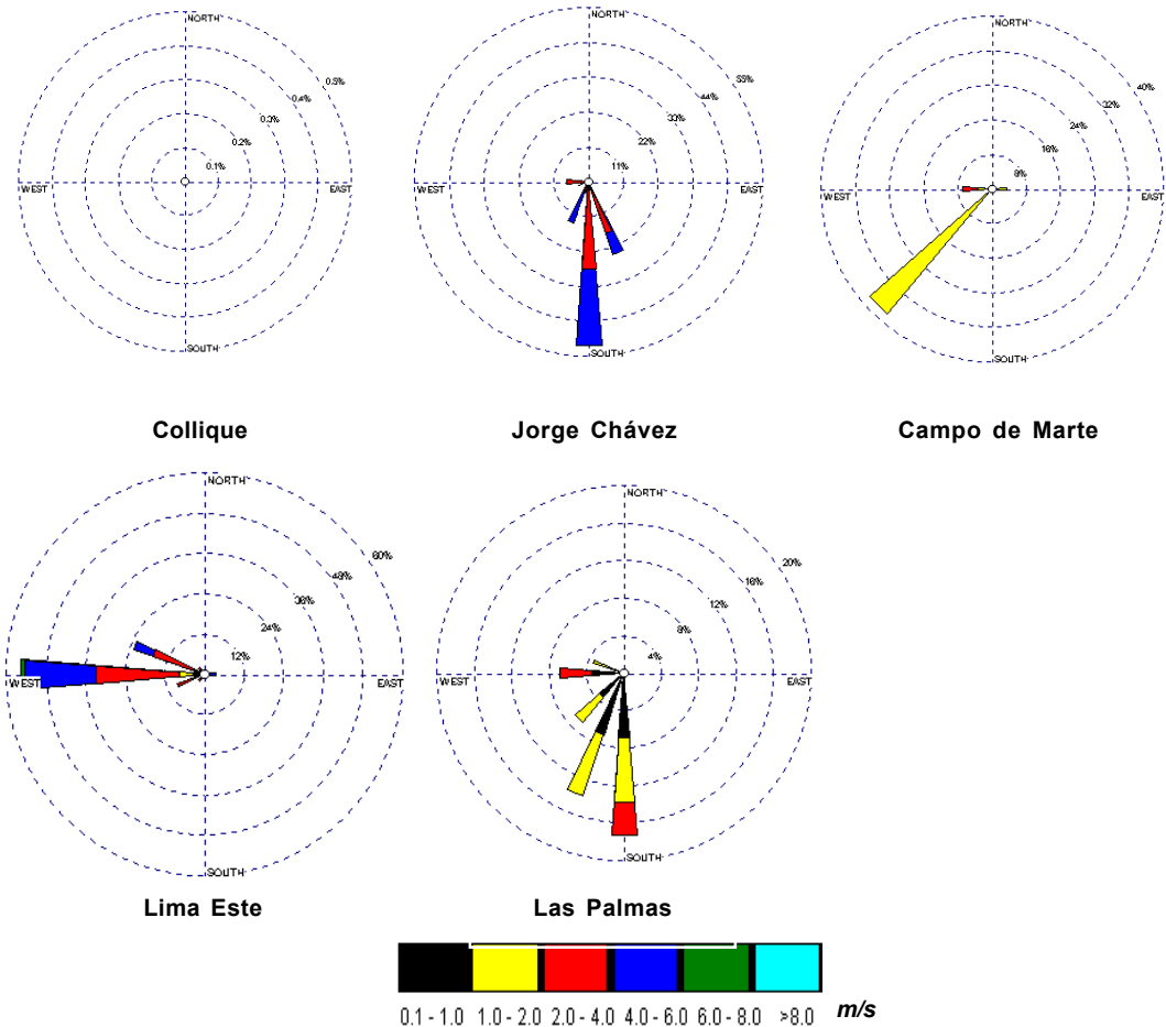
Figura 6. Rosas de viento (m/s) de las 07:00 horas de estaciones meteorológicas
