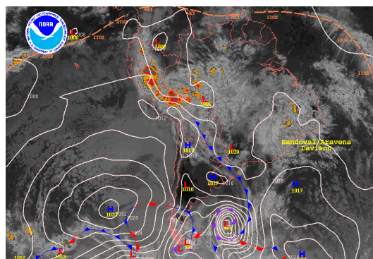
Figura 7. Imagen satelital del día 29 de diciembre del 2003.
