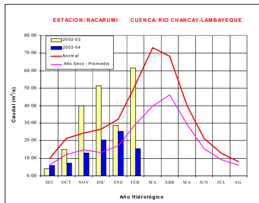
Gráfico 4. Caudal medio mensuales del año hidrológico 2002-2003, 2003-2004, año promedio o Normal y año seco promedio del río Chancay-Lambayeque
