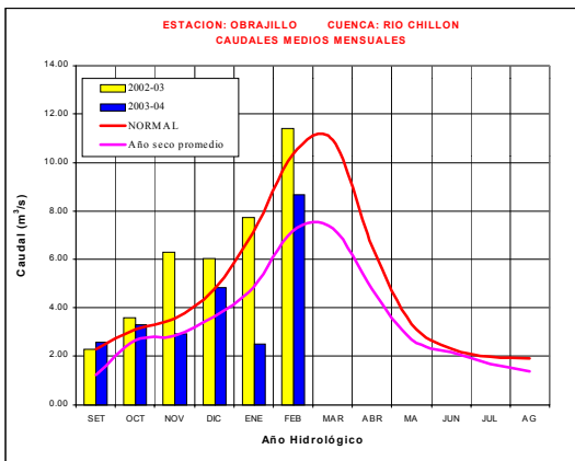
Gráfico 6. Caudales medios mensuales del año hidrológico 2002-2003, 2003-2004, año promedio o normal y año seco promedio del río Chillón
