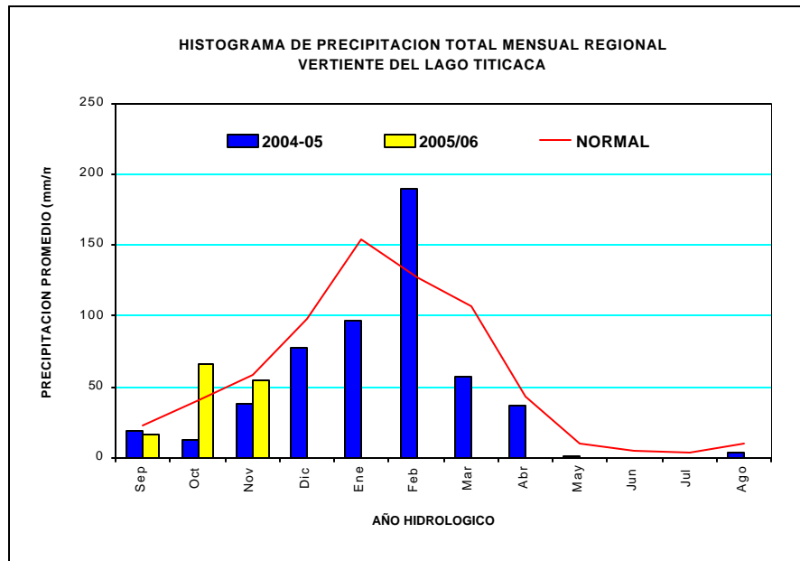
GRÁFICO 10: HISTOGRAMA DE PRECIPITACIÓN TOTAL MENSUAL REGIONAL DE LA VERTIENTE DEL LAGO TITICACA
