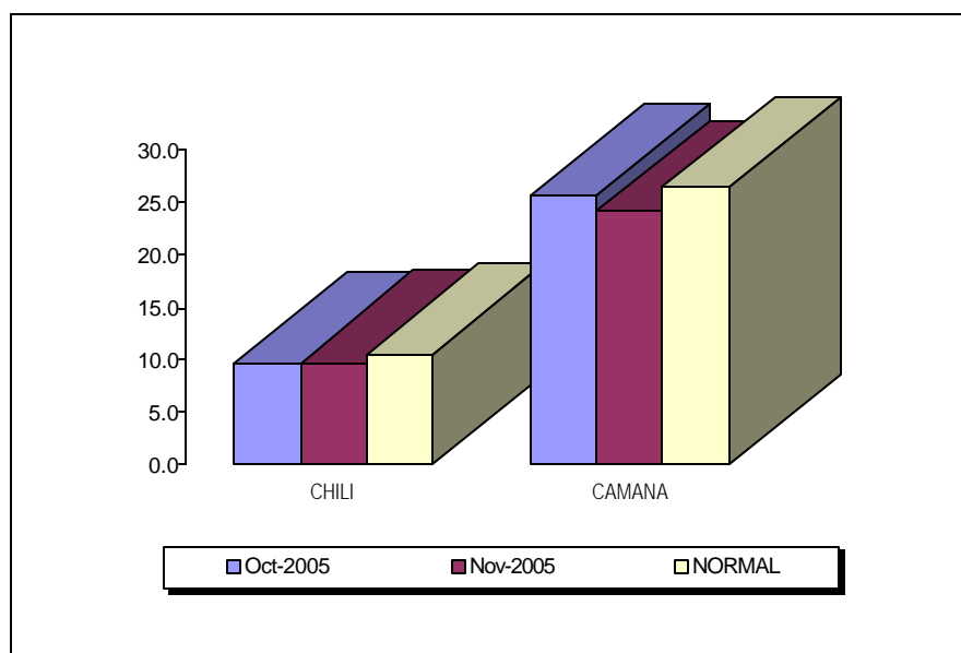
GRÁFICO N° 7: HISTOGRAMA DE LOS CAUDALES MEDIOS MENSUALES POR CUENCAS DE LOS RÍOS DE LA VERTIENTE DEL OCÉANO PACÍFICO - ZONA SUR
