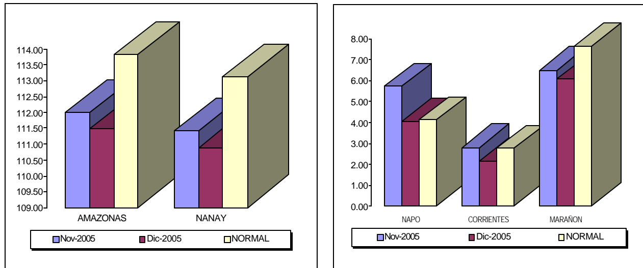
FIGURA Nº 16: HISTOGRAMA DE PRECIPITACIÓN TOTAL MENSUAL POR CUENCAS DE LA VERTIENTE DEL ATLÁNTICO - ZONA CENTRAL
