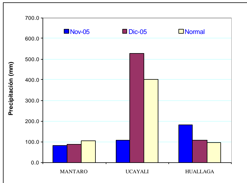
FIGURA Nº 16: HISTOGRAMA DE PRECIPITACIÓN TOTAL MENSUAL POR CUENCAS DE LA VERTIENTE DEL ATLÁNTICO - ZONA CENTRAL
