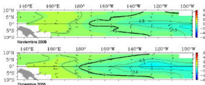
Fig. 1. Anomalia de la temperatura superficial del mar (°C) 10°N-10°S
