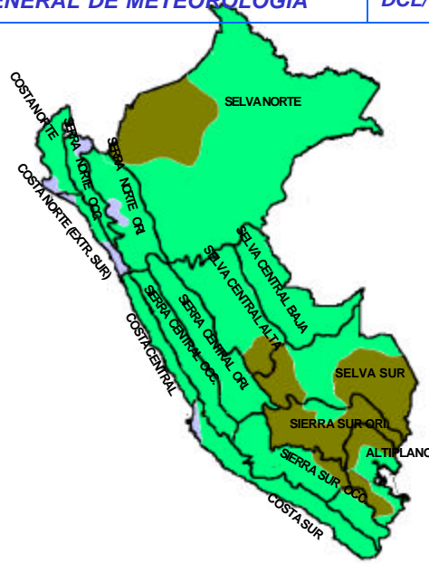
PROBABILIDAD DE OCURRENCIA DE TEMPERATURAS MINIMAS DEL AIRE PERIODO: ENERO-MARZO 2006
