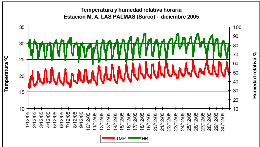
Fig.5a.- Variación horaria de la temperatura y humedad relativa durante el mes de diciembre del 2005 en Comas, El Callao y Santiago de Surco
