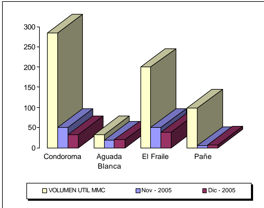
FIGURA Nº 24: VOLUMEN ALMACENADOS EN LOS RESERVORIOS DE LA ZONA SUR
