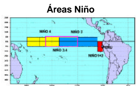
Fig. 2 : Temperatura Superficial del Mar en áreas Niño
