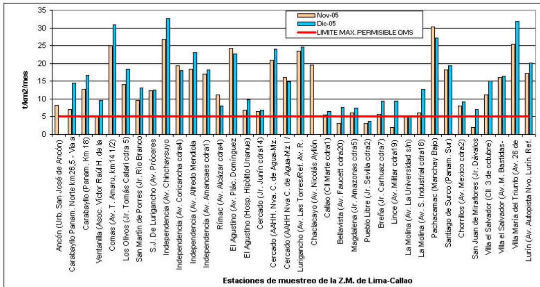
Fig.2-Totales mensuales de polvo atmosférico (contaminantes sólidos sedimentables) registrados durante los meses de noviembre y diciembre 2005 en Lima-Callao
