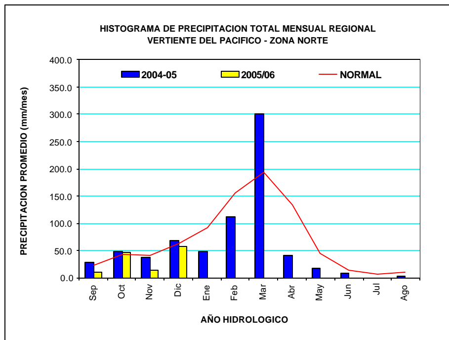
FIGURA Nº 2: HISTOGRAMA DE PRECIPITACIÓN TOTAL MENSUAL REGIONAL DE LA VERTIENTE DEL OCEANO PACÍFICO - ZONA NORTE
