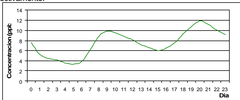
Fig.4e -. Concentración máxima media horaria de dióxido de nitrógeno Estación de calidad de aire SENAMHI - diciembre 2005
