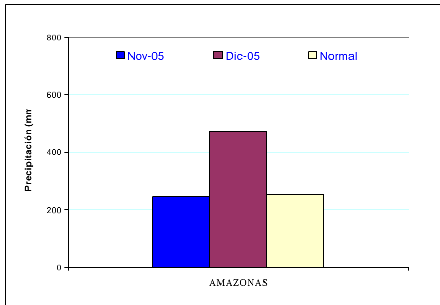
FIGURA Nº 14: HISTOGRAMA DE PRECIPITACIÓN TOTAL MENSUAL REGIONAL DE LA VERTIENTE DEL ATLÁNTICO – ZONA NORTE
