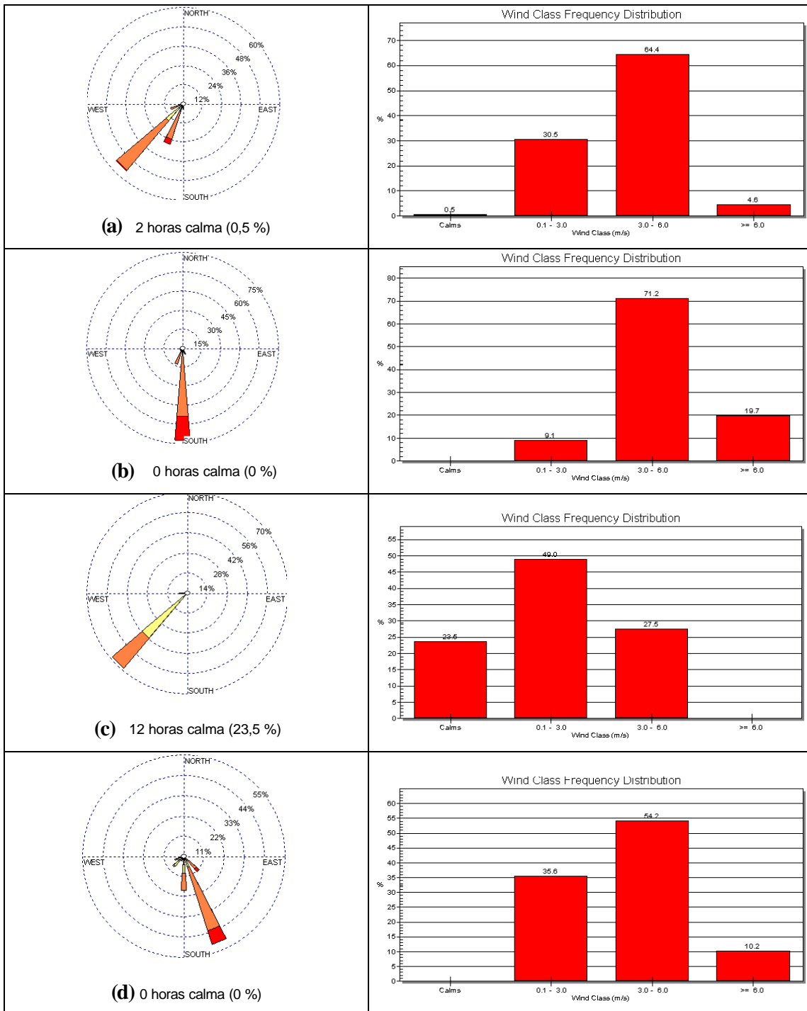
Fig. 6. Rosa de viento diurnas de las estaciones de a) Comas b) Callao c) J. María d) Surco. Diciembre 2005
