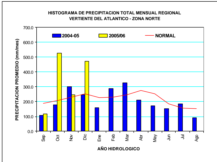
FIGURA Nº 13: HISTOGRAMA DE PRECIPITACIÓN TOTAL MENSUAL POR CUENCA DE LA VERTIENTE DEL ATLÁNTICO – ZONA NORTE
