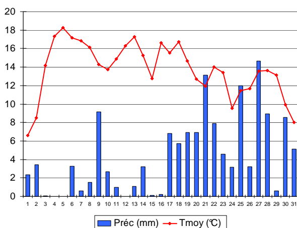
Figure 1a : Températures moyennes et précipitations journalières de mai 2006 à l'échelle nationale
