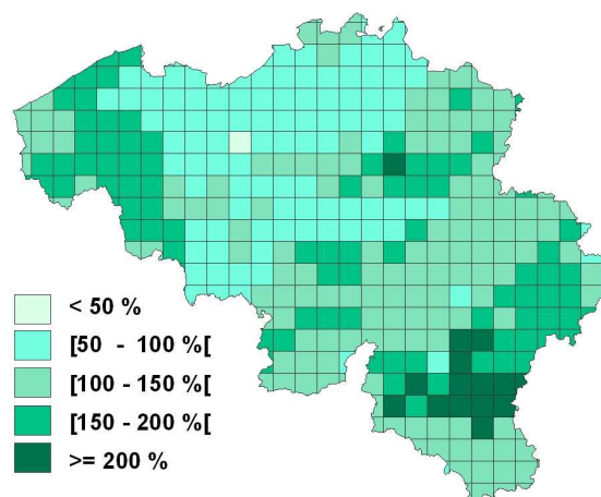
Figure 1b : Ecart en %, des précipitations de mai 2006 par rapport à la moyenne (1988-2005)
