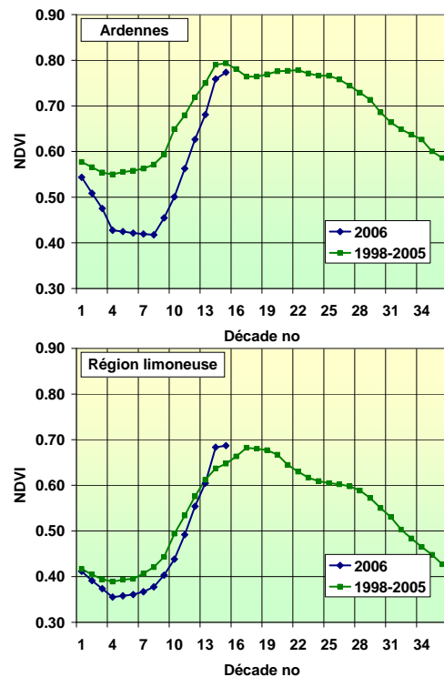
Figure 3 - [a] Écart relatif (%) de l'état de la végétation (NDVI, dérivé d'images satellitaires SPOT-VEGETATION) pour la période de janvier à mai 2006 par rapport à la moyenne historique (1998-2005) et [b] évolution de la végétation (reflétée par le NDVI) par rapport à la moyenne historique pour les Ardennes et la Région limoneuse.
