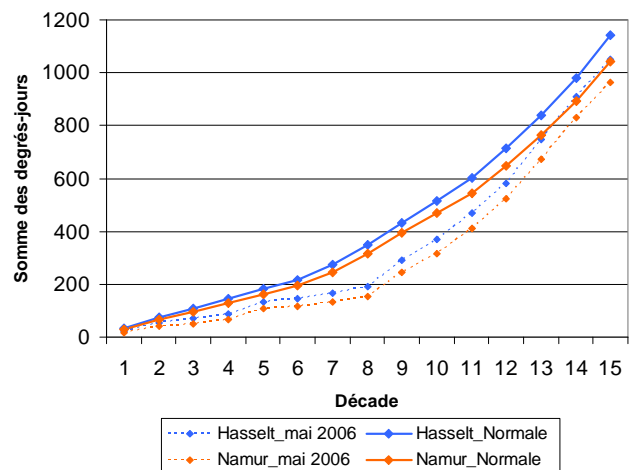
Figure 2b : Somme des degrés-jours depuis le 1.1.2006 pour les régions de Hasselt et Namur ; valeurs 2006 en pointillé et moyennes en continu
