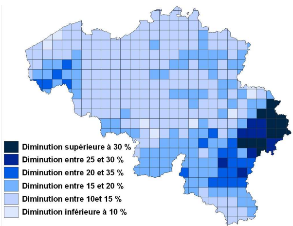
Figure 2a : Ecart de la somme des degrés-jours par rapport à la moyenne (1988-2005)
