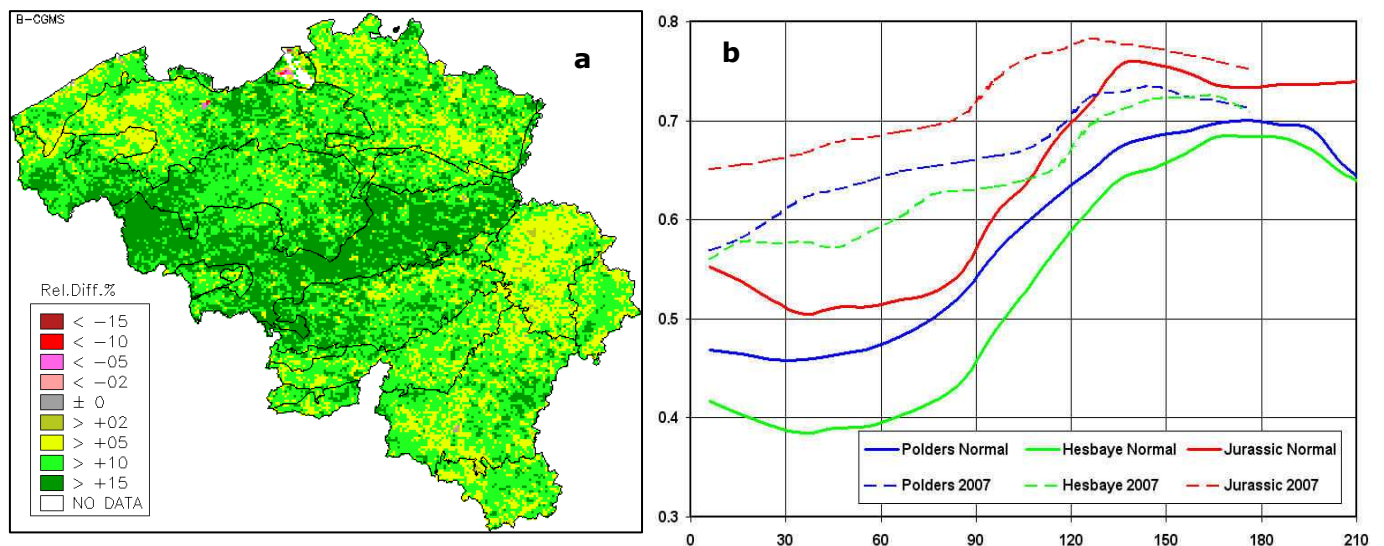
Figure 2: [a] Écart relatif (%) de l'état de la végétation (NDVI, dérivé d'images satellitaires SPOT-VEGETATION) pour la période Mars-Juin 2007 par rapport à la moyenne historique (1988-2006, "Normale") et [b] évolution de la végétation (NDVI en fonction des jours) pour les mêmes trois régions que dans la figure 1.
