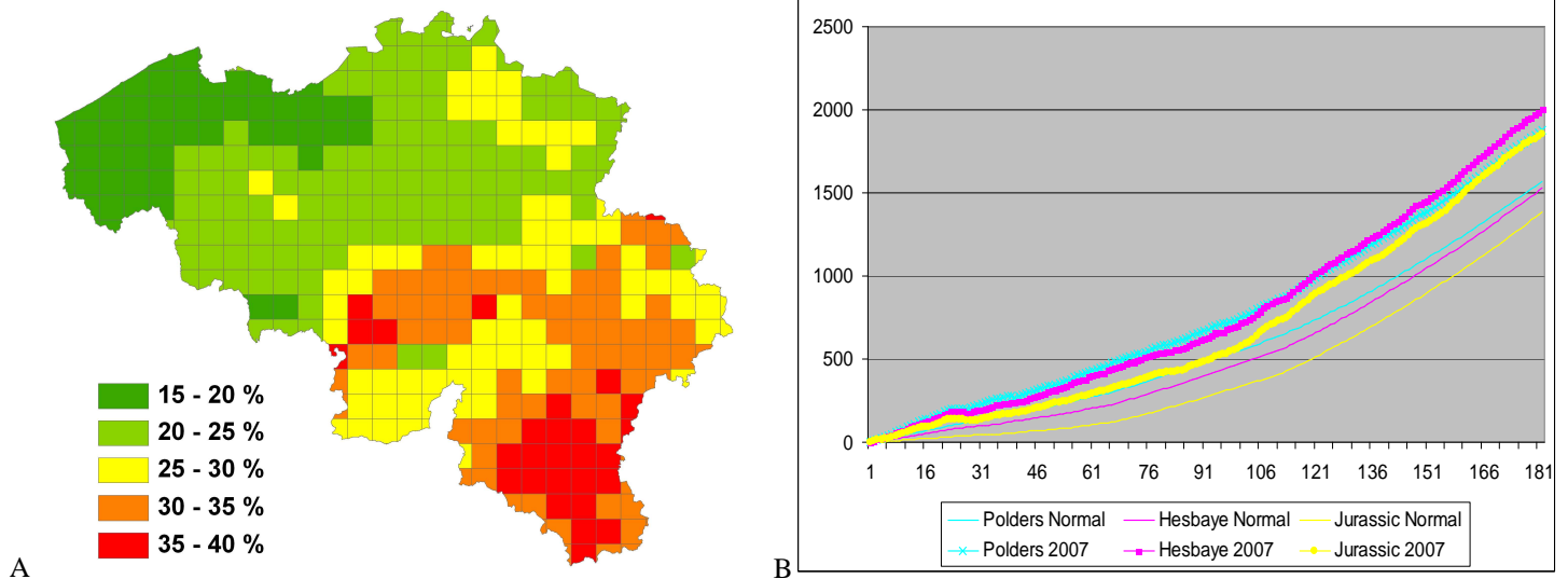
Figure 1 : (a) Ecart (%) de la somme des degrés.jours entre le 1.1 et le 30.6.2007 par rapport à la normale calculée sur la période 1988-2006. (b) Evolution des sommes de degrés.jours(°C) en 2007 et en situation normale pour trois régions du nord, centre et sud du pays
