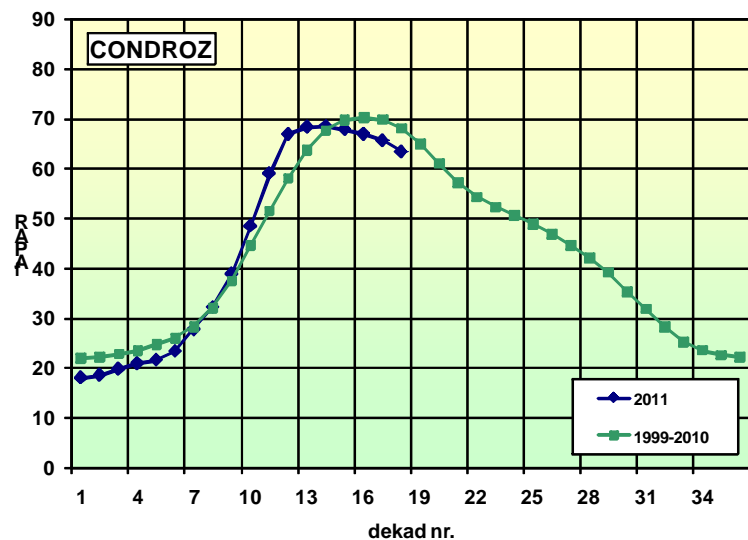
Figure 3 : Profils d’évolution de l’indice de végétation de janvier à juin: 2011 et moyenne 1999-2010 pour [a] la Région Sablonneuse et [b] le Condroz
