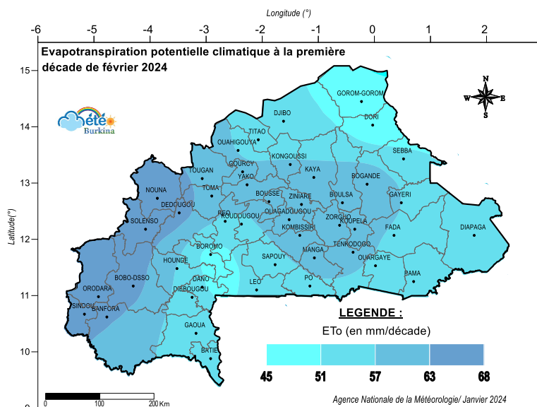
Figure o : Prévision climatologique de l'ETP à la première décennie de février 2024
