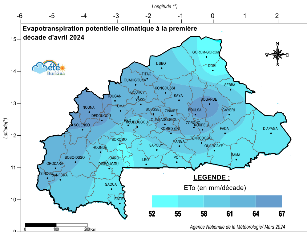
Figure o : Prévision climatologique de l'ETP à la première décennie d'avril 2024
