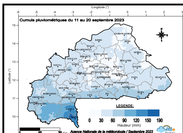
Figure 1 : Cumuls pluviométriques à la deuxième décennie de septembre 2023.
