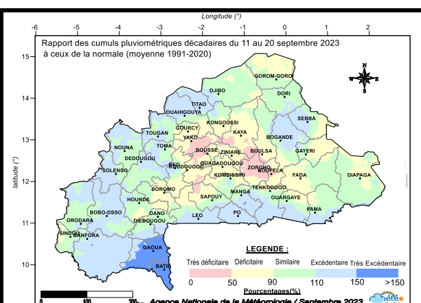
Figure 2 : Rapport des cumuls pluviométriques à la deuxième décennie de septembre 2023 à la normale 1991-2020.
