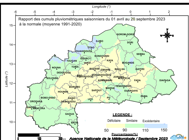
Figure 4 : Rapport des cumuls pluviométriques du 01 avril au 20 septembre 2023 à la normale 1991-2020.
