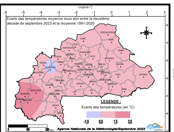
Figure 7 : Ecart des températures moyennes sous abri entre la deuxième décennie de septembre 2023 et la moyenne (1991-2020).
