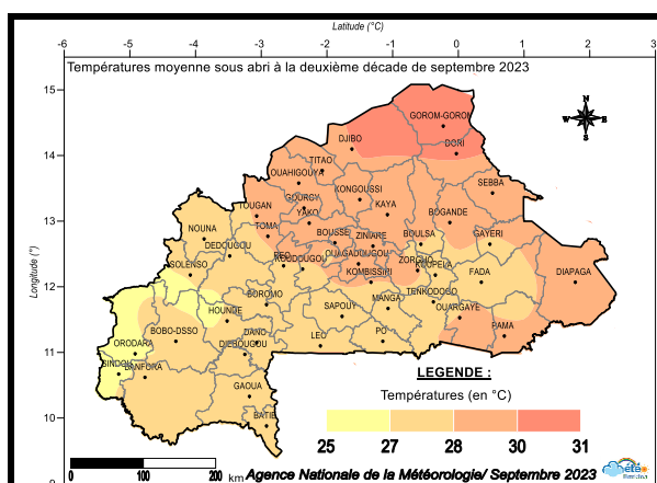
Figure 6 : Températures moyennes sous abri à la deuxième décennie de septembre 2023.
