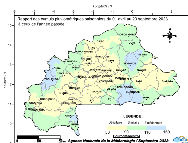
Figure 5 : Rapport des cumuls pluviométriques du 1 er avril au 20 septembre 2023 à ceux de l'année précédente.
