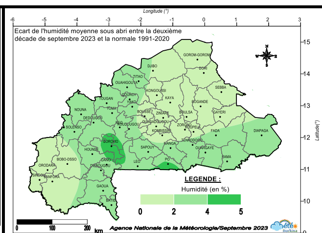
Figure 9 : Ecart de l'humidité relative moyenne entre la deuxième décennie de septembre 2023 et la moyenne (1991-2020).
