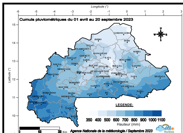
Figure 3 : Cumuls pluviométriques saisonniers du 01 avril au 20 septembre 2023.
