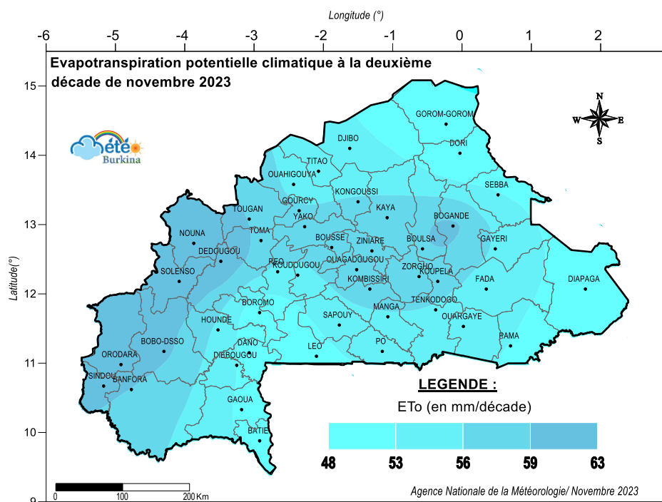
Figure o : Prévision climatologique de l’ETP à la deuxième décennie de novembre 2023
