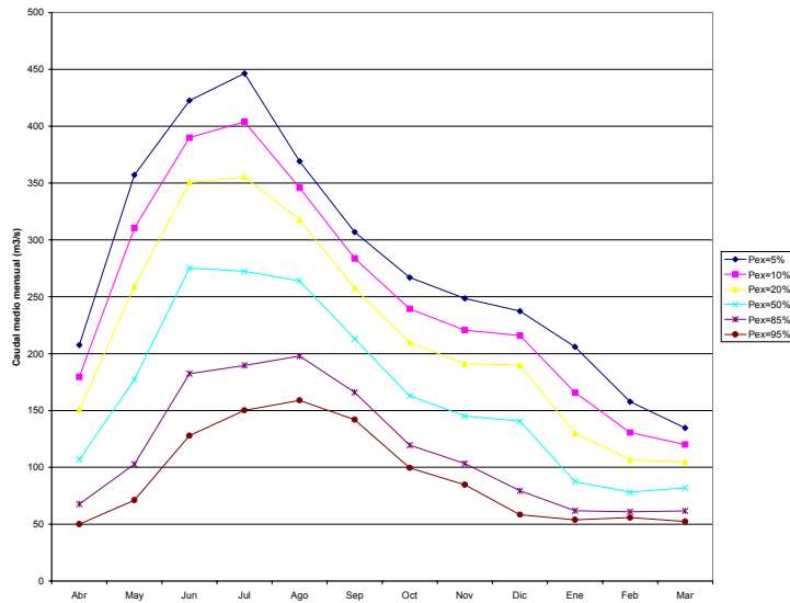
Figura 4.4: Curva de Variación Estacional Río Pilmaiquén en San Pablo
