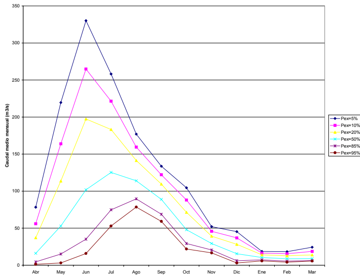
Figura 4.8: Curva de Variación Estacional Río Negro en Chahuilco
