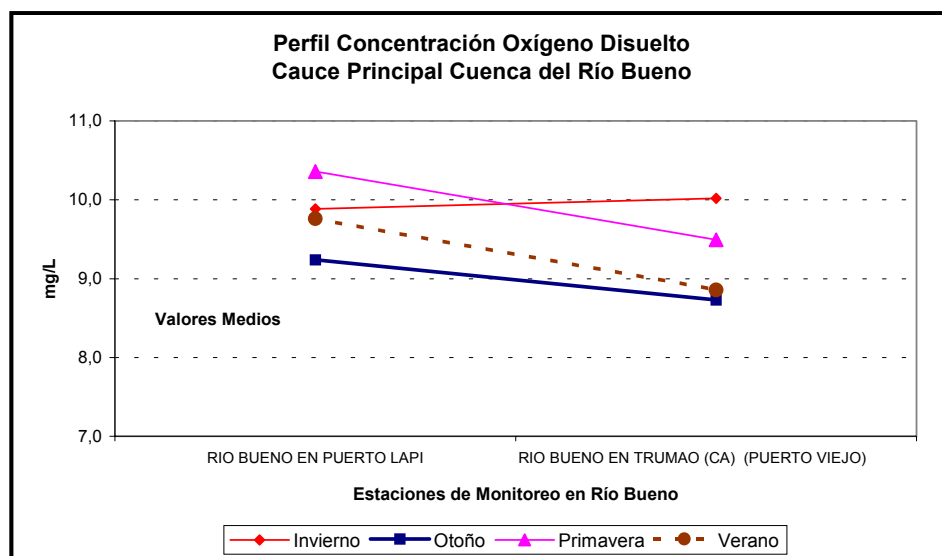
Figura 5.1: Perfil Longitudinal de Calidad de Agua en la Cuenca de Río Bueno
