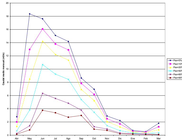
Figura 4.7: Curva de Variación Estacional Río Forrahue en Aromos
