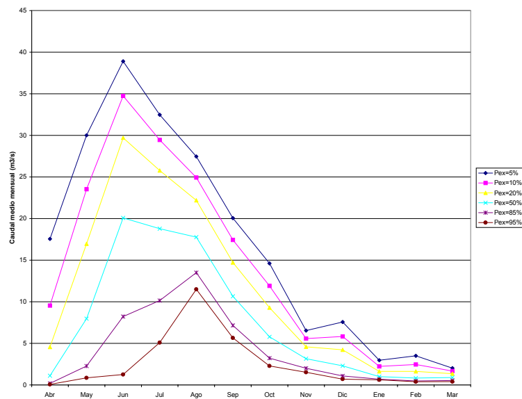
Figura 4.9: Curva de Variación Estacional Río Damas en Tacamo
