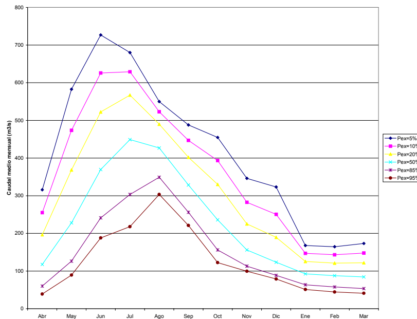
Figura 4.10: Curva de Variación Estacional Río Rahue en Forrahue
