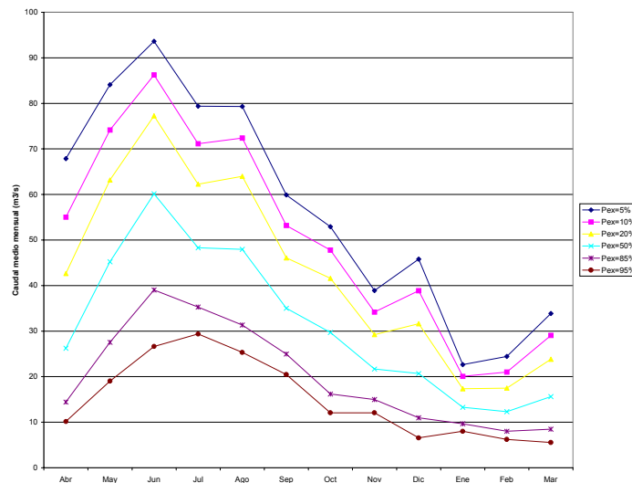
Figura 4.6: Curva de Variación Estacional Río Coihueco antes junta Pichicope
