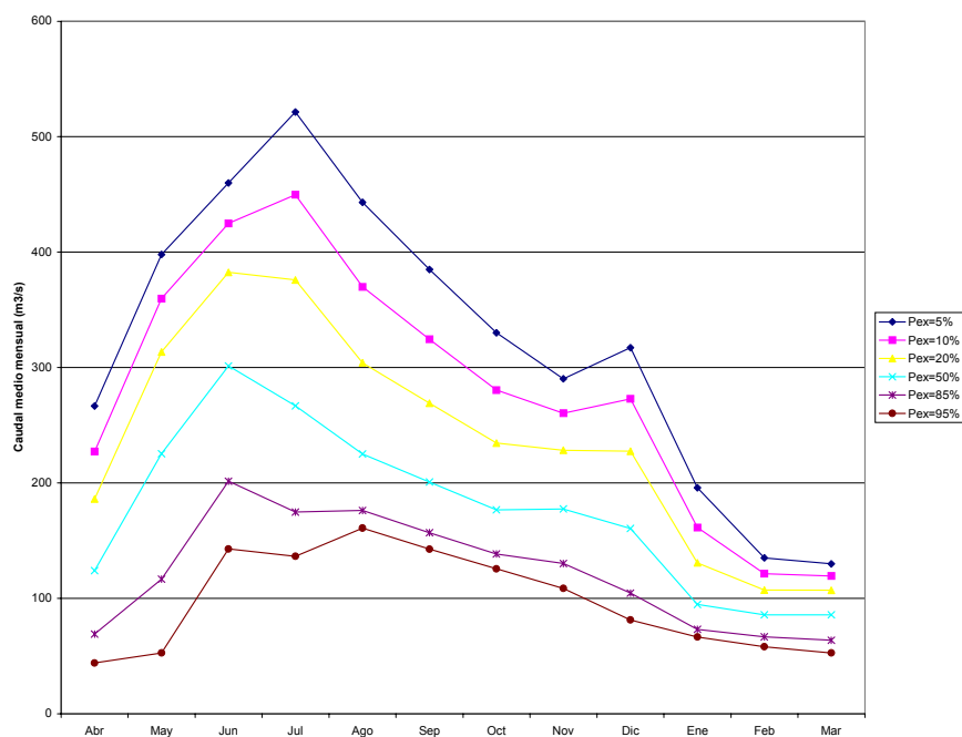
Figura 4.1: Curva de Variación Estacional Río Calcarrupe en desembocadura
