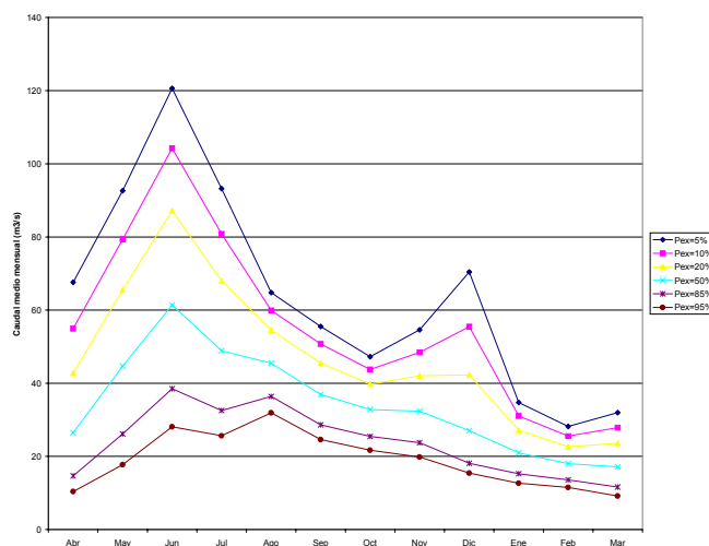
Figura 4.2: Curva de Variación Estacional Río Nilahue en Mallay
