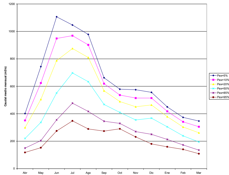
Figura 4.3: Curva de Variación Estacional Río Bueno en Bueno
