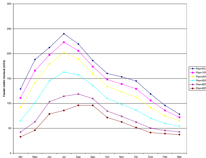
Figura 4.5: Curva de Variación Estacional Río Rahue en desagüe lago Rupanco
