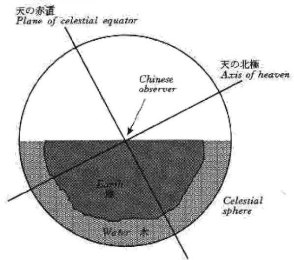
図 3.5 渾天説
