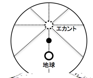
図 4.3 エカント
