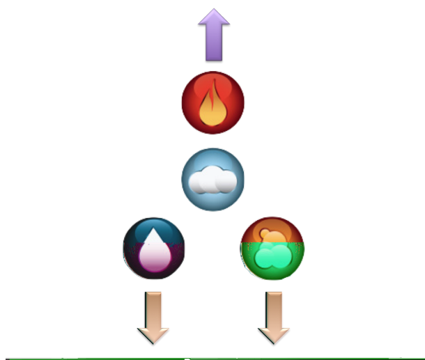
図 1.5 物質の本性
