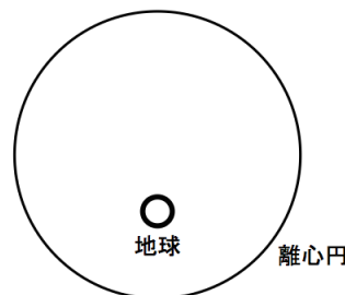
図 4.2 離心円
