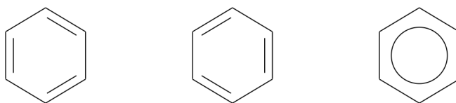
図 10.4 ベンゼン
