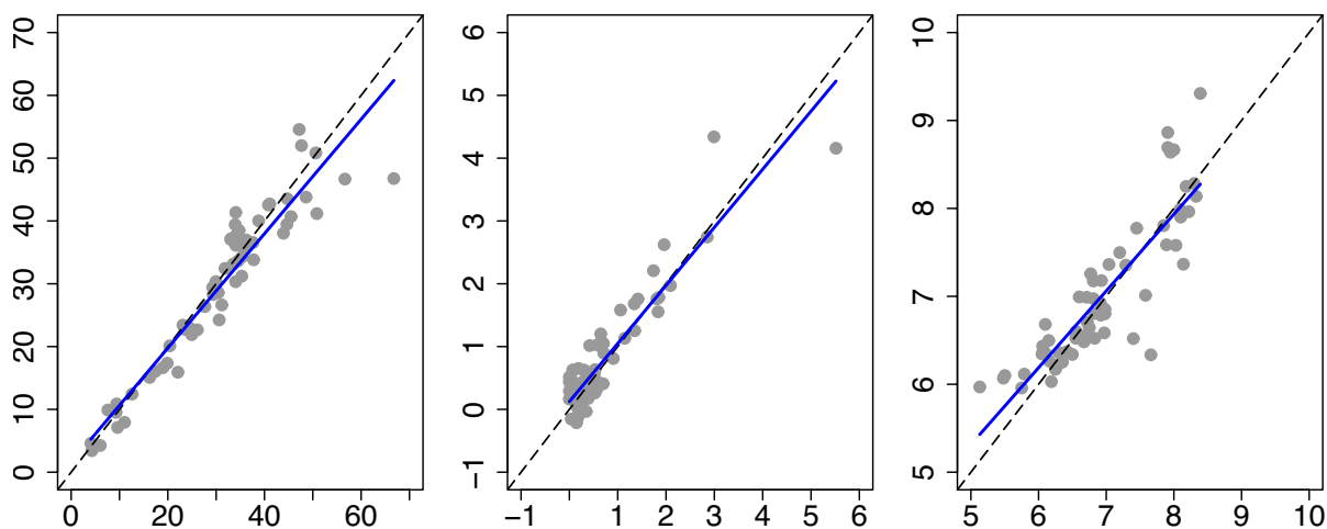
Figure 7. Diagrammes de dispersion des propriétés du sol prédites par le système vis-NIR et mesurées en laboratoire pour le jeu de données test (n = 60) à l'aide de la régression partielle par les moindres carrés. La ligne grise en pointillés est une ligne d'égalité entre le mesuré au laboratoire et le prédit, tandis que la ligne bleue est la ligne ajustée aux mesures. Source : Auteurs du présent document
