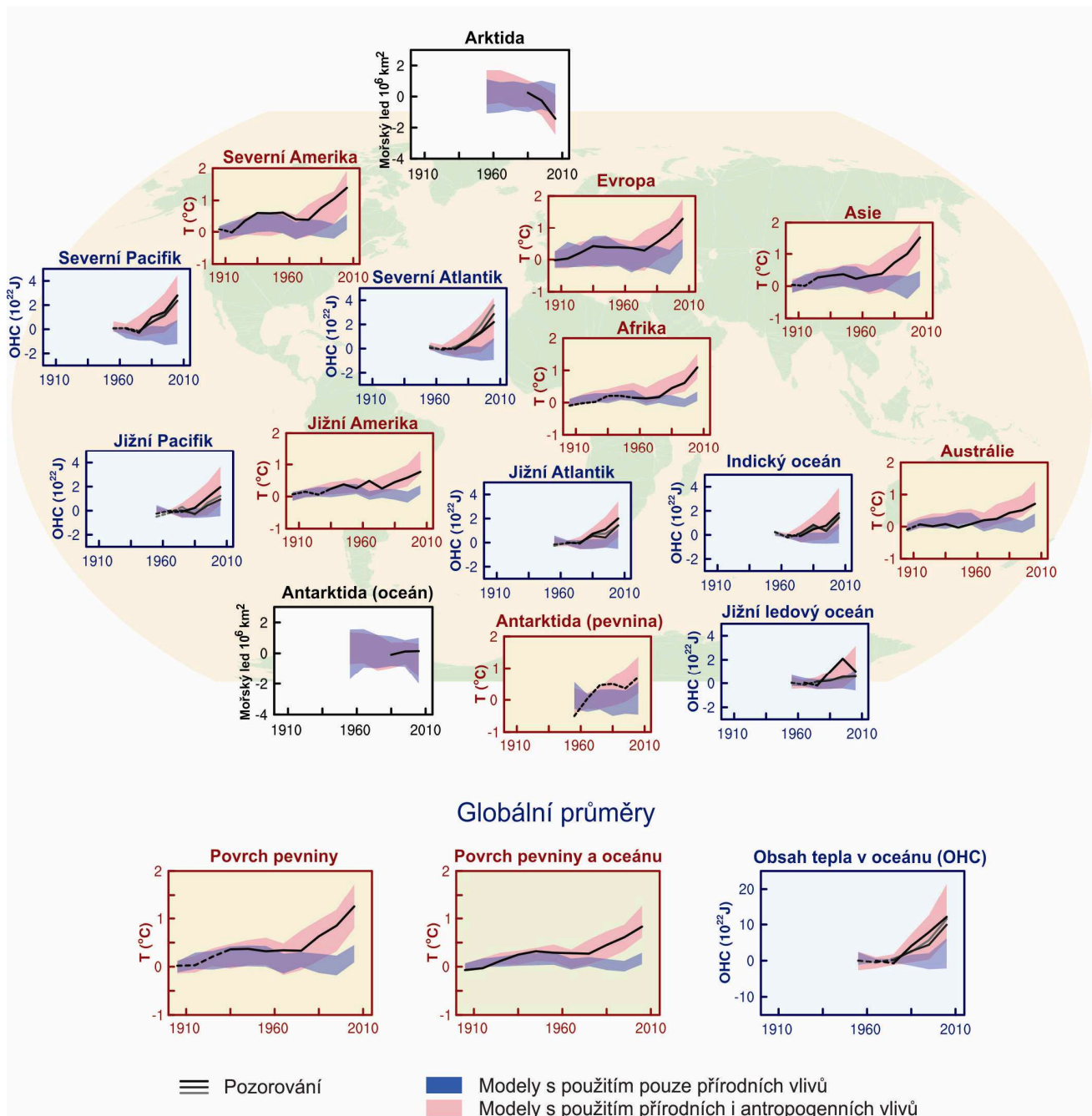
Obr. SPM.6: Srovnání pozorované a simulované změny klimatu na základě tří velkoprostorových indikátorů v atmosféře, kryosféře a oceánu: změna teploty vzduchu při povrchu nad kontinenty (žluté panely), rozsah arktického a antarktického mořského ledu v září (bílé panely) a obsah tepla ve vrchních vrstvách oceánu ve velkých oceánských pánvích (modré panely). Uvedeny jsou také globální průměrné změny. Anomálie jsou uvedeny vzhledem k období 1880-1919 u teploty vzduchu při povrchu, 1960-1980 u obsahu tepla v oceánu a 1979-1999 u mořského ledu. Všechny časové řady jsou průměry za desetiletí vyznačené ke středě dekad. U teplotních panelů jsou pozorování vyznačena přerušovanou čarou, pokud prostorové pokrytí zkoumaných oblastí bylo pod 50 %. U panelů znázorňujících obsah tepla v oceánu a mořský led je použita plná čára tam, kde je dobré datové pokrytí a vyšší kvalita dat a přerušovaná čára je tam, kde je datové pokrytí jen dostatečné a neurčitost je tedy větší. Znázorněné výsledky modelů jsou rozsahy ansámbly z multimodelových výstupů z projektu CMIP5, kde vystínovaná pásma označují intervaly spolehlivosti 5 až 95 %. Další odborné informace, včetně definic oblastí, jsou uvedeny v Dodatku k Technical Summary (obr. 10.21; obr. TS.12)
