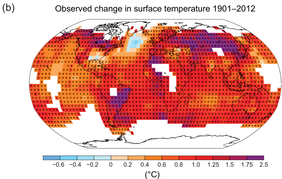
Figuur SPM. 1 | (a) Waargenomen wereldwijd gemiddelde gecombineerde land en zee temperatuur anomalieën, voor 1850 tot 2012 volgens drie datasets. Bovenste paneel: jaargemiddelde waarden, onderste paneel: 10 jaargemiddelde waarden inclusief een schatting van de onzekerheid voor één dataset (zwart). Anomalieën zijn ten opzichte van het gemiddelde voor 1961–1990. (b) Kaart van de waargenomen veranderingen in oppervlaktetemperatuur in de periode 1901–2012 afgeleid uit temperatuurtrends verkregen door lineaire regressie van één dataset (oranje lijn in paneel a). De trends zijn berekend waar voldoende data beschikbaar zijn voor een robuuste schatting (dat wil zeggen alleen voor roostercellen met meer dan 70% data beschikbaarheid en meer dan 20% data beschikbaarheid in de eerste en laatste 10% van de periode). Andere gebieden zijn wit. Roostercellen waar de trend significant is op een niveau van 10% zijn aangegeven met een + teken.
