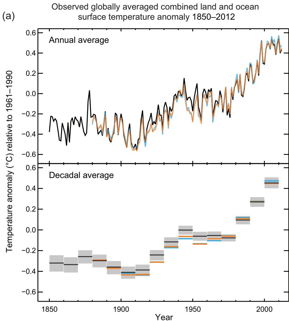
Figuur SPM. 1 | (a) Waargenomen wereldwijd gemiddelde gecombineerde land en zee temperatuur anomalieën, voor 1850 tot 2012 volgens drie datasets. Bovenste paneel: jaargemiddelde waarden, onderste paneel: 10 jaargemiddelde waarden inclusief een schatting van de onzekerheid voor één dataset (zwart). Anomalieën zijn ten opzichte van het gemiddelde voor 1961–1990. (b) Kaart van de waargenomen veranderingen in oppervlaktetemperatuur in de periode 1901–2012 afgeleid uit temperatuurtrends verkregen door lineaire regressie van één dataset (oranje lijn in paneel a). De trends zijn berekend waar voldoende data beschikbaar zijn voor een robuuste schatting (dat wil zeggen alleen voor roostercellen met meer dan 70% data beschikbaarheid en meer dan 20% data beschikbaarheid in de eerste en laatste 10% van de periode). Andere gebieden zijn wit. Roostercellen waar de trend significant is op een niveau van 10% zijn aangegeven met een + teken.
