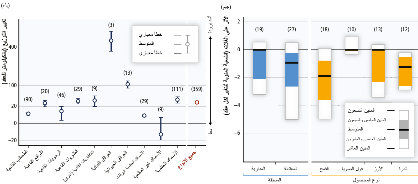
الشكل SPM.2 | الآثار الواسعة النطاق في عالم متغير. (ألف) الأنماط العالمية للآثار في العقود الأخيرة المعزوة إلى تغير المناخ، استناداً إلى الدراسات التي أجريت منذ تقرير التقييم الرابع. والآثار مبنية على مدى النطاقات الجغرافية. وتشير الرموز إلى فئات الآثار المعزوة، والمساهمة النسبية لتغير المناخ (الرئيسي أو الطفيف) في الآثار الملحوظة، والثقة في العزو. انظر الجدول التكميلي SPM.A1 للاطلاع على أوصاف الآثار. (باء) متوسط معدلات التغير في التوزيع (بالكيلومتر للعدد) بالنسبة لمجموعات الأنواع البحرية استناداً إلى رصدات على مدى الفترة 2010-1900. والتغيرات الإيجابية في التوزيع تتسق مع الاحترار (الانتقال إلى مياه كانت أشد برودة سابقاً، في اتجاه القطب عموماً). ويبين عدد الاستجابات المحللة الوارد بين أقواس لكل فئة. ملخص الآثار المقدرة لتغيرات المناخ الملحوظة على الغلات خلال الفترة 2013-1960 بخصوص أربعة محاصيل رئيسية في مناطق معتدلة ومناطق مدارية، مع تبيان عدد نقاط البيانات المحللة بين أقواس فيما يتعلق بكل فئة. [الأشكال 2-7 و 2-18 و 3-2 و MB-2]
