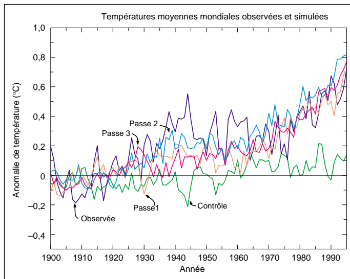
Figure TS 13 — Anomalies des températures (°C) moyennes mondiales observées et simulées, par rapport à la moyenne des observations pour la période 1900 à 1930. Les données de contrôle et les trois simulations indépendantes effectuées avec le même gaz à effet de serre accompagné d'un forçage d'aérosols, dans des conditions initiales légèrement différentes, sont tirées d'un modèle AOGCM. Les trois simulations sont identifiées comme "passe 1", "passe 2" et "passe 3" respectivement.
