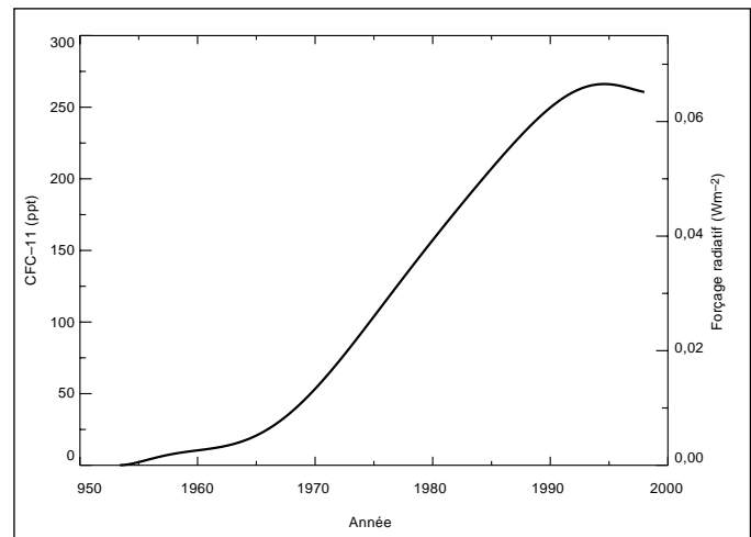
Figure TS 12 — Concentration moyenne mondiale (ppt) de CFC-11 (CFC13) dans la troposphère, de 1950 à 1998, déterminée à partir de mesures lissées et de modèles d'émission. Le forçage radiatif du CFC-11 est indiqué sur l'axe de droite.
