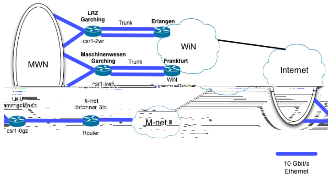
Abbildung 8: Redundante Internet-Anbindung über X-WiN und M-net
