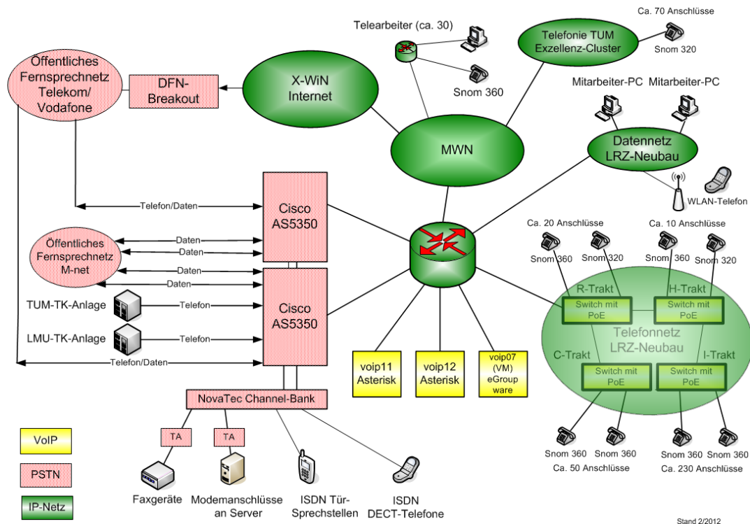
Abbildung 12: VoIP-TK-Anlage am LRZ
