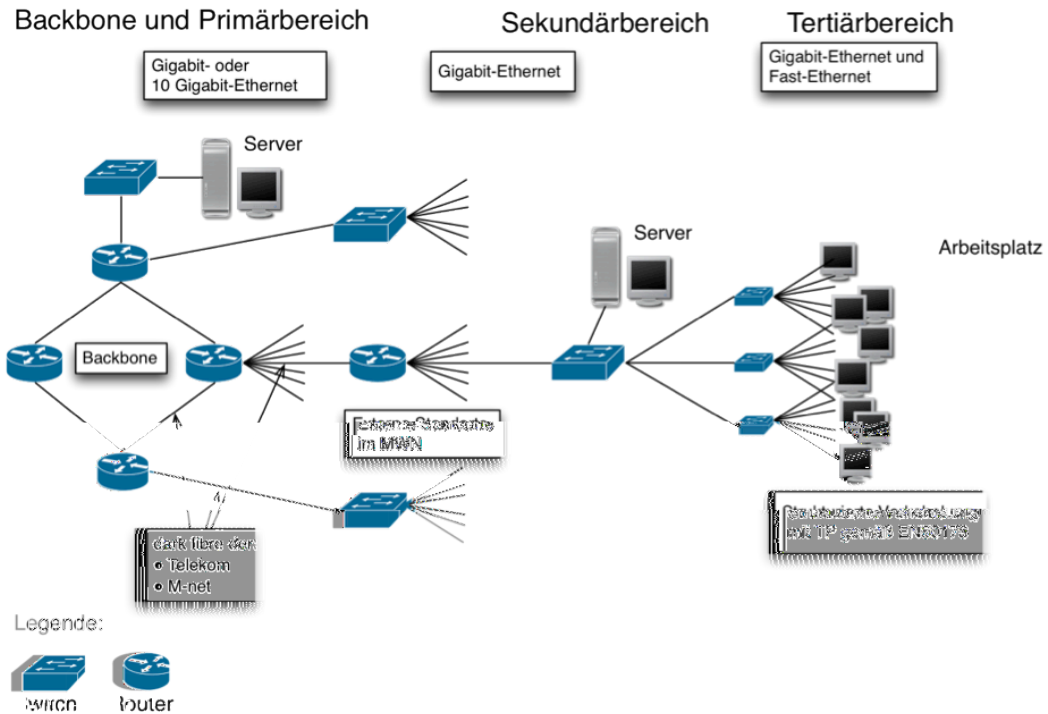
Abbildung 7: Schematische Verkabelungsstruktur
