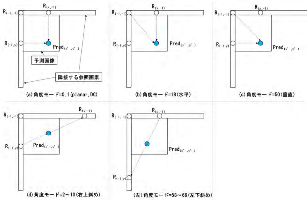
図 4-8 PDPC の各予測モードにおける隣接参照画素
