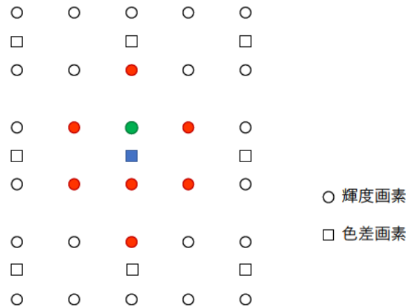
図 7-9 CC-ALF のフィルタ処理に用いる画素位置
