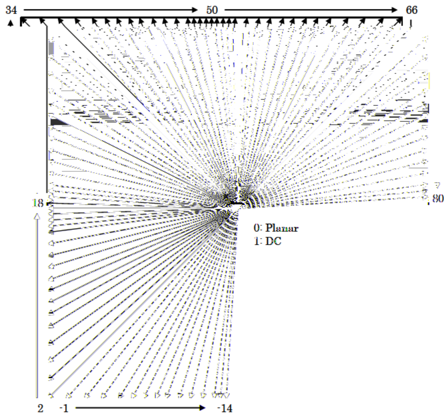
図 4-1 予測ブロックと隣接参照画素
