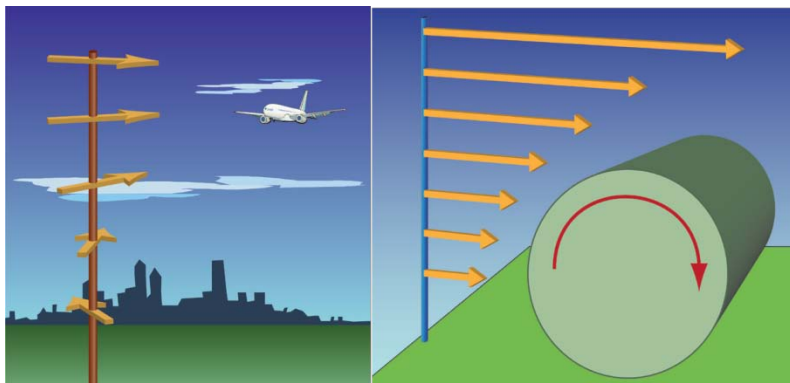
Unos ejemplos de la cizalladura direccional (izq.) y cizalladura por velocidad (der.)
