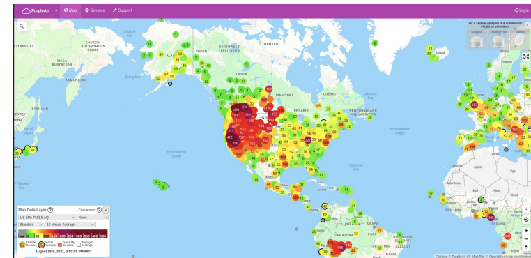
Dust/Aerosol Data
