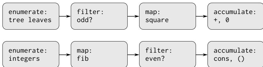
図 2.7: 手続き sum-odd-squares (上) と even-fibs (下) を信号の流れという図式によって表現すると、二つのプログラムの共通性が明らかになる。
