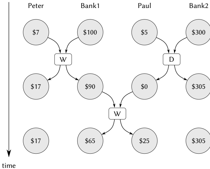
図 3.30: 銀行 1 の共同口座と銀行 2 の個人口座に対する並行な預け入れと引き出し
