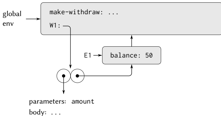
図 3.9: W1 呼び出し後の環境
