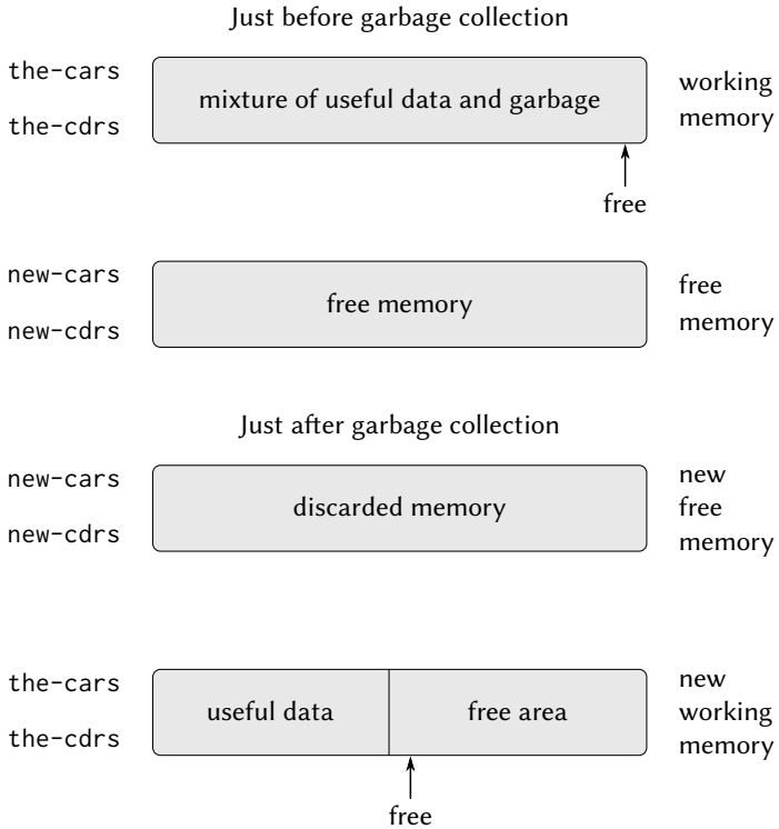
図 5.15: ガベージコレクション処理によるメモリの再構成
