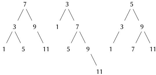
図 2.16: 集合 \{1, 3, 5, 7, 9, 11\} を表現するさまざまな二分木
