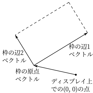
図 2.15: 枠は、原点と二つの辺という三つのベクトルによって記述される。
