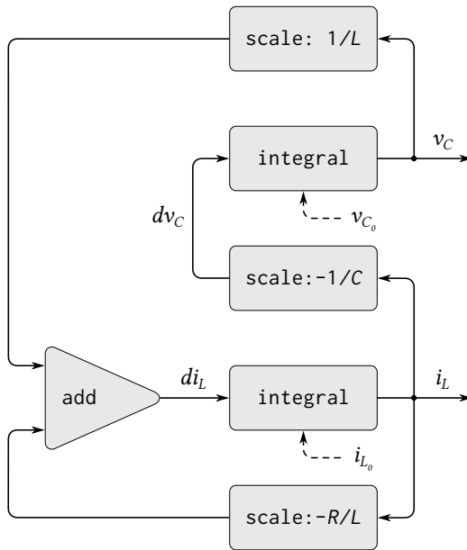
図 3.37: 直列 RLC 回路を解くための信号フロー図
