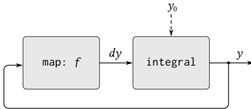
図 3.34: 方程式 dy/dt = f(y) を解く “アナログ計算回路”
