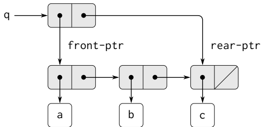
図 3.19: 先端と終端のポインタを持つリストとしてのキューの実装
