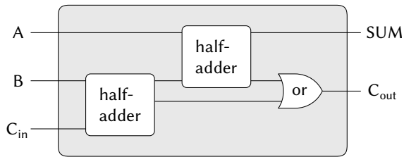
図 3.26: 全加算器回路
