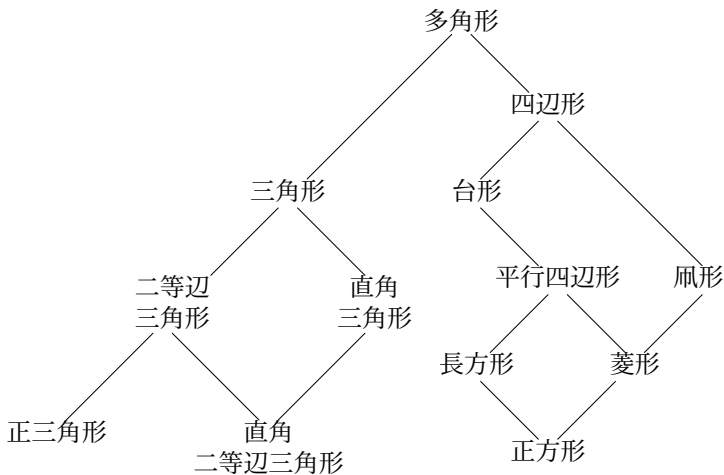
図 2.26: 幾何学図形の型の間関係
