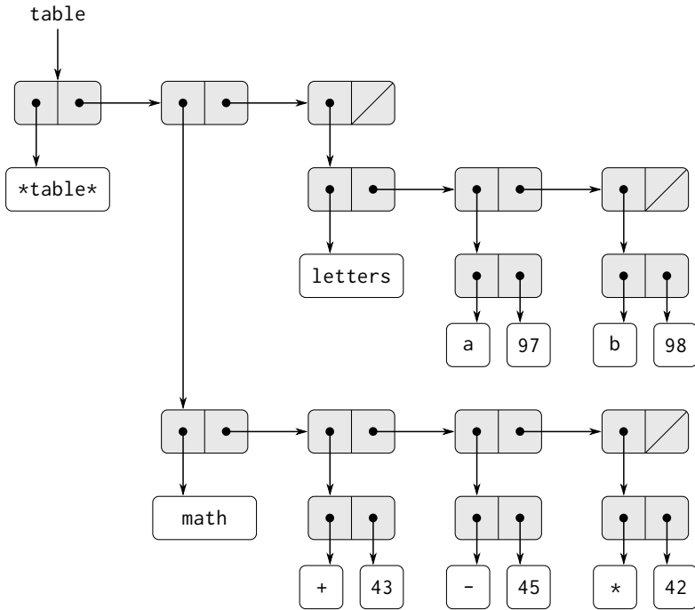
図 3.23: 二次元テーブル
