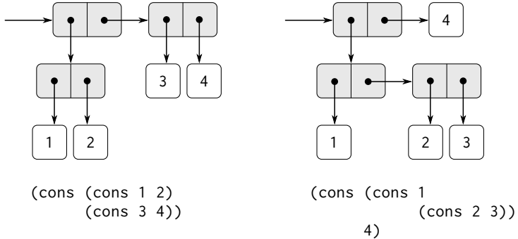
図 2.3: ペアを使って 1, 2, 3, 4 を組み合わせる二つの方法
