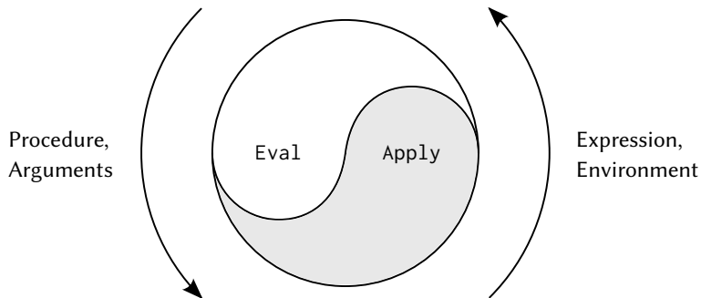
図 4.1: eval-apply サイクルが明らかにするコンピュータ言語の本質
