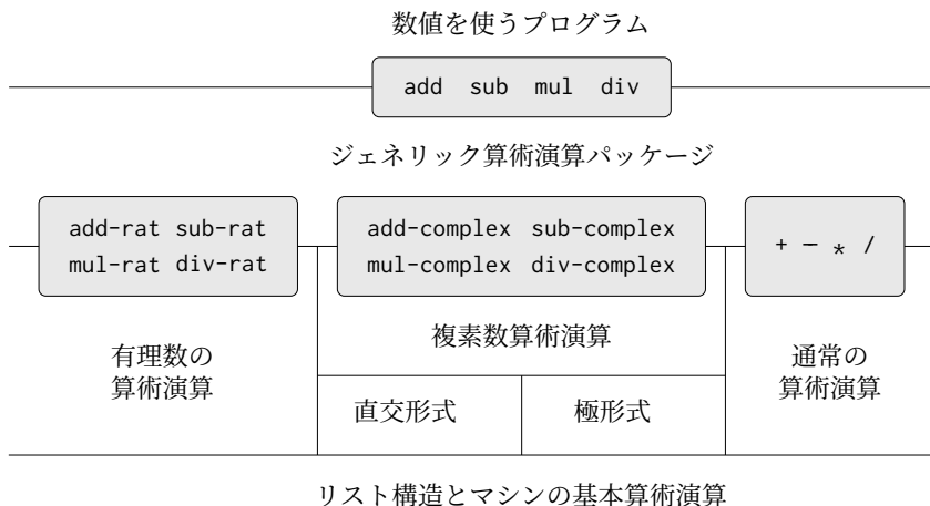
図 2.23: ジェネリック算術演算システム
