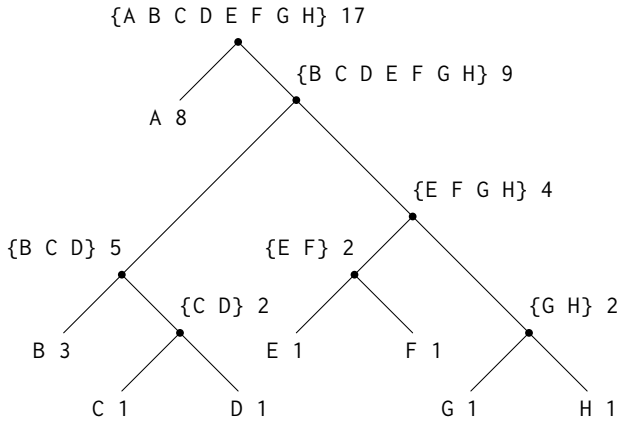
図 2.18: ハフマン符号化木
