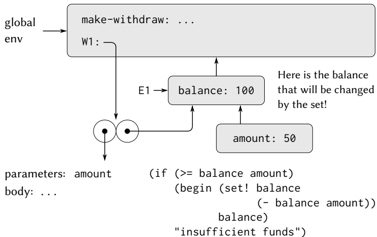
図 3.8: 手続きオブジェクト W1 を適用することによって作成される環境
