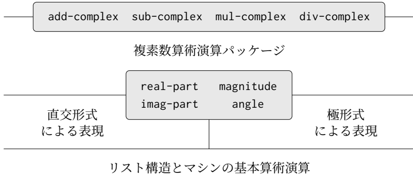
図 2.21: ジェネリックな複素数算術演算システムの構造
