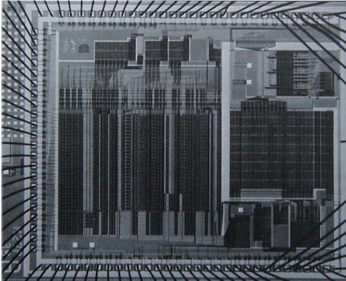
図 5.16: Scheme 評価器のシリコンチップ実装
