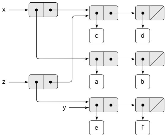
図 3.14: 図 3.12 のリストに対する (define z (cons y (cdr x))) の効果
