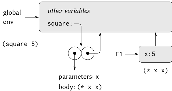
図 3.3: グローバル環境で (square 5) を評価することによって作られる環境
