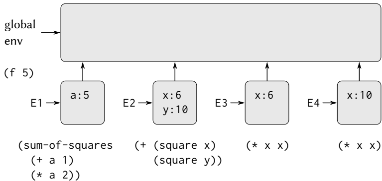
図 3.5: 図 3.4内の手続きを用いて (f 5) を評価することで作られた環境
