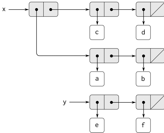
図 3.12: リスト x: ((a b) c d) と y: (e f)
