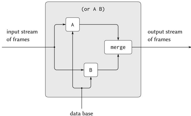
図 4.6: 二つのクエリの or による組み合わせは、フレームのストリームに対して並列に演算を行い、その結果をマージすることによって生成される
