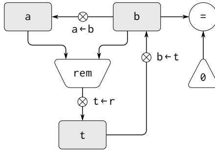
図 5.1: GCD マシンのデータパス
