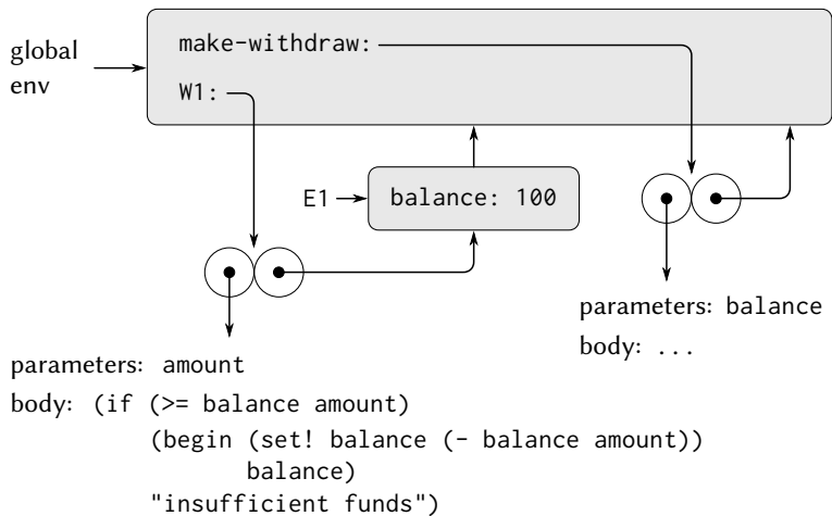
図 3.7: (define W1 (make-withdraw 100)) を評価した結果
