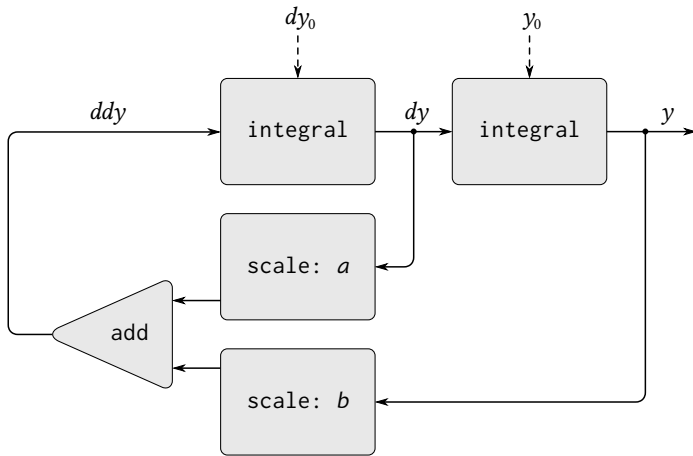
図 3.35: 二次線形微分方程式を解くための信号フロー図
