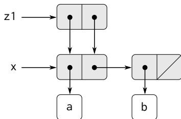
図 3.16: (cons x x) によって作られるリスト z1
