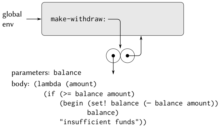
図 3.6: グローバル環境で make-withdraw を定義した結果
