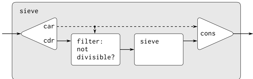
図 3.31: 信号処理システムとして見た素数のふるい
