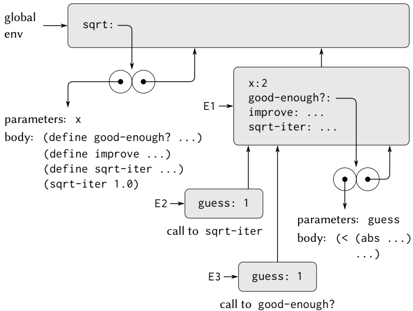
図 3.11: 内部定義を持つ sqrt 手続き
