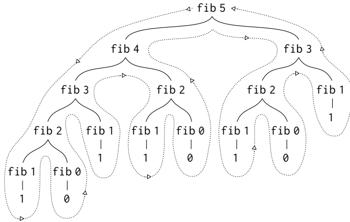
図 1.5: (fib 5) の計算時に生成される木の再帰プロセス
