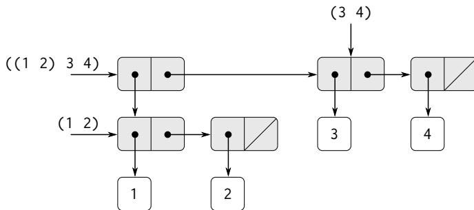
図 2.5: (cons (list 1 2) (list 3 4)) によって作られる構造
