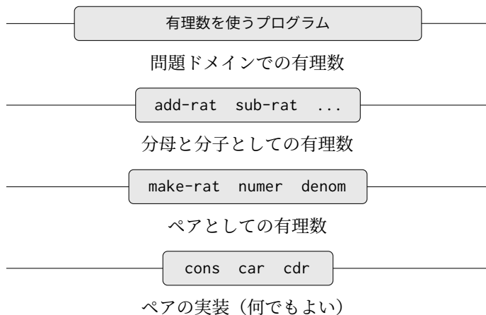
図 2.1: 有理数パッケージ内の抽象化の壁
