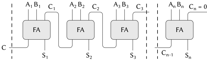
図 3.27: n bit の数を扱う繰り上がり伝播加算器
