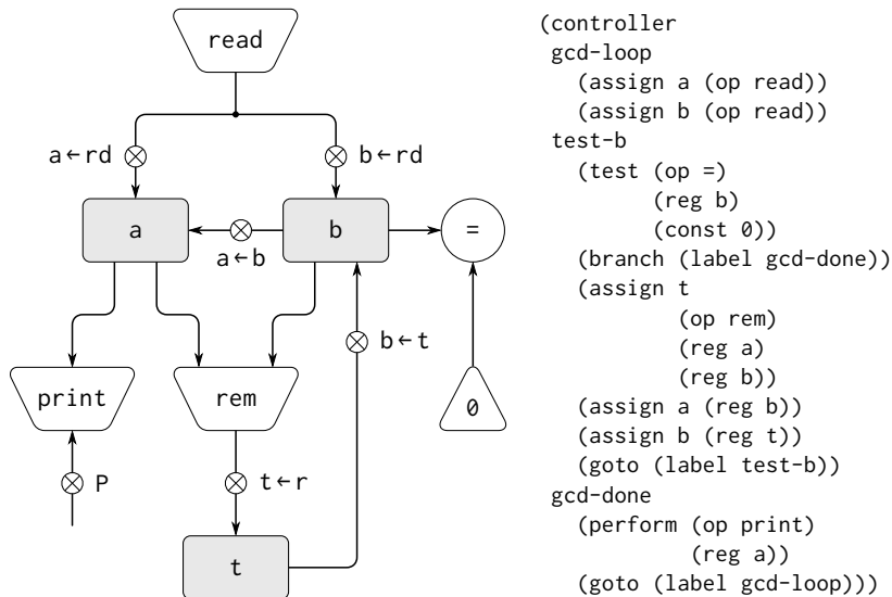
図 5.4: 入力を読み込み結果を表示する GCD マシン
