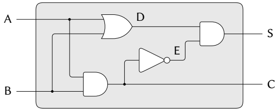
図 3.25: 半加算器回路
