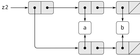
図 3.17: (cons (list 'a 'b) (list 'a 'b)) によって作られるリスト z2
