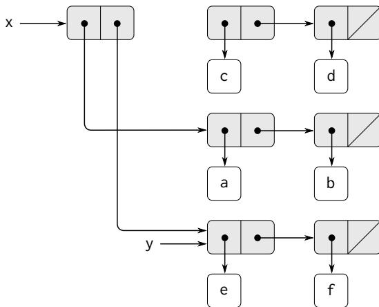
図 3.15: 図 3.12 のリストに対する (set-cdr! x y) の効果
