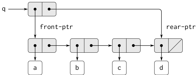
図 3.20: 図 3.19のキューに (insert-queue! q 'd) を使った結果
