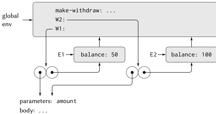
図 3.10: (define W2 (make-withdraw 100)) を使って二つ目のオブジェクトを作成
