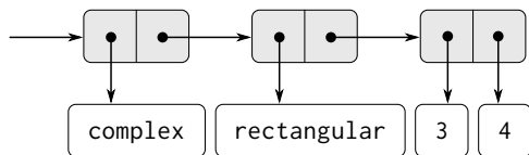
図 2.24: 直交形式による 3 + 4i の表現
