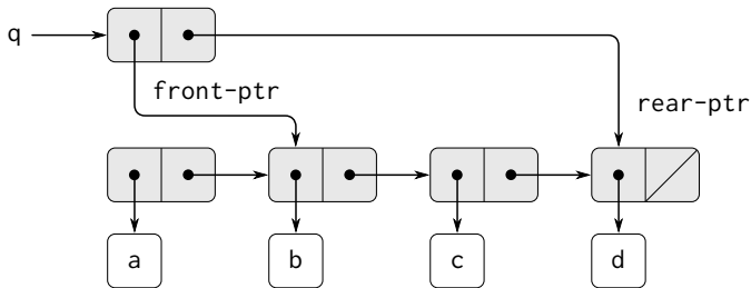
図 3.21: 図 3.20のキューに (delete-queue! q) を使った結果
