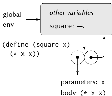
図 3.2: グローバル環境の中で (define (square x) (* x x)) を評価することによって作られる環境
