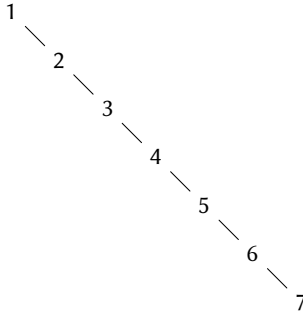
図 2.17: 1 から 7 まで順番に追加するとできるバランスの取れていない木
