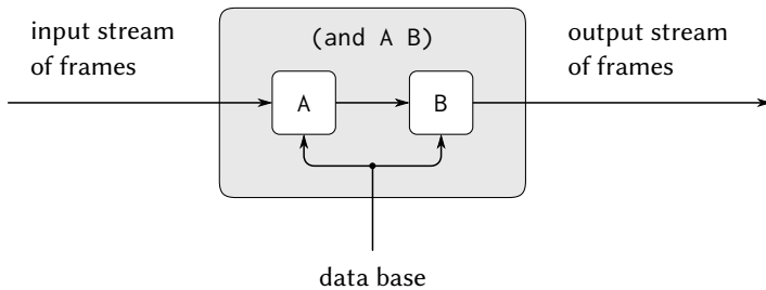
図 4.5: 二つのクエリの and による組み合わせは、フレームのストリームに対する直列の演算によって生成される
