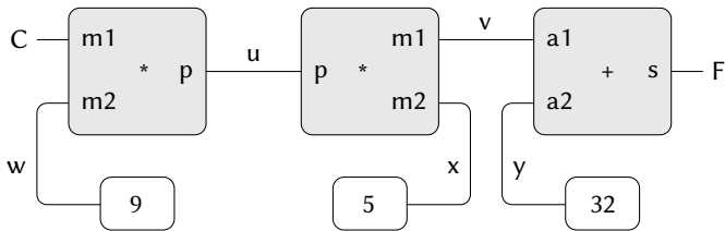
図 3.28: 制約ネットワークとして表現された関係 9C = 5(F - 32)
