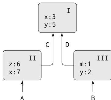
図 3.1: 単純な環境構造
