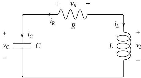
図 3.36: 直列 RLC 回路
