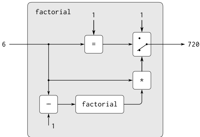
図 4.2: 抽象機械として見た階乗プログラム
