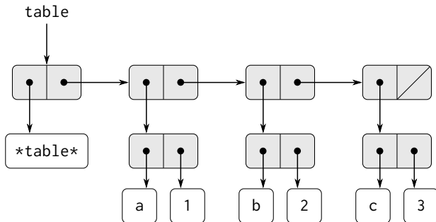
図 3.22: 頭つきリストとして表現されたテーブル
