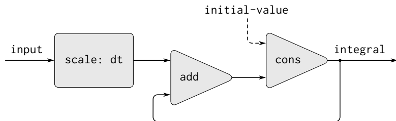
図 3.32: 信号処理システムとして見た integral 手続き
