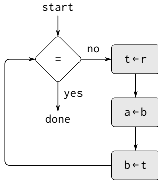
図 5.2: GCD マシンのコントローラ
