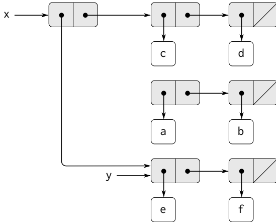
図 3.13: 図 3.12 のリストに対する (set-car! x y) の効果
