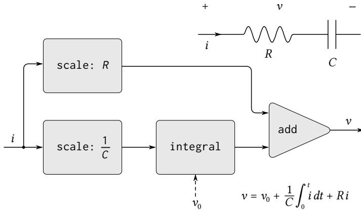
図 3.33: RC 回路と対応する信号流れ図
