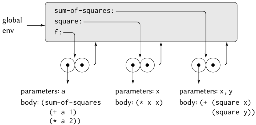
図 3.4: グローバルフレーム内の手続きオブジェクト
