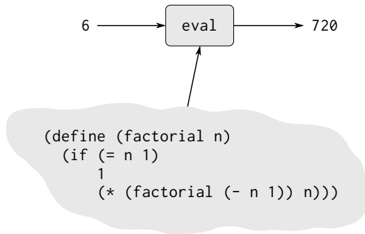
図 4.3: 階乗マシンの動作を模倣する評価器
