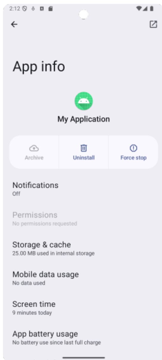
図 4.1.8 Force stop
