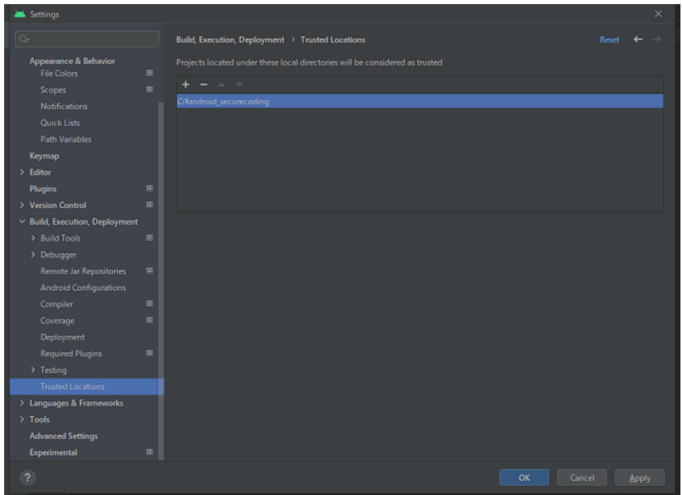
図 2.5.23 C:\android_securecoding を追加
