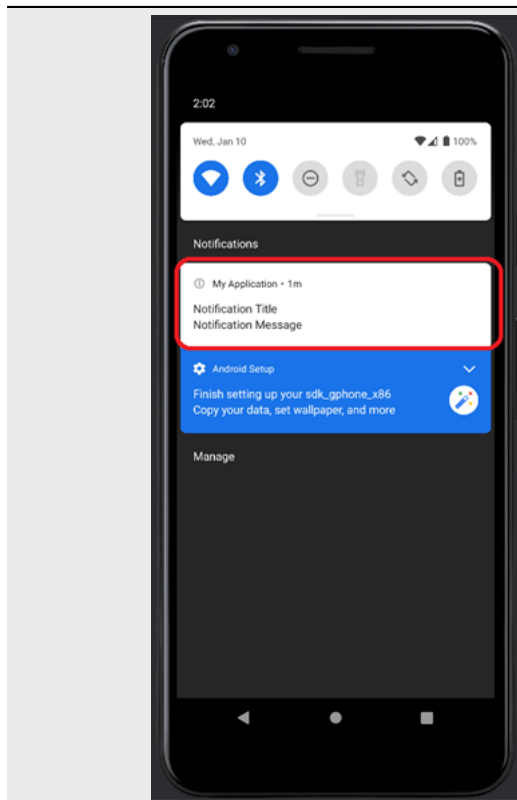
図 4.10.9 Android 11 の Notification
