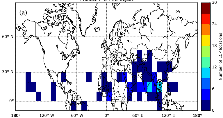
Phase1 &gt; 8 PVU EQLat
