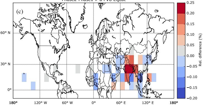
Phase2-Phase1 &gt; 8 PVU EQLat
