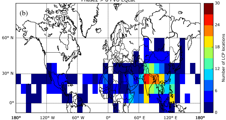
Phase2 &gt; 8 PVU EQLat
