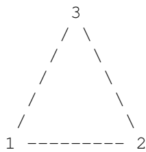
ESMF_MESHELEMENTTYPE_TRI
