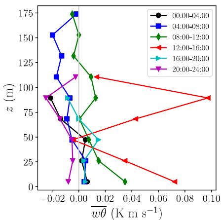
(d) Vertical kinematic sensible heat flux
